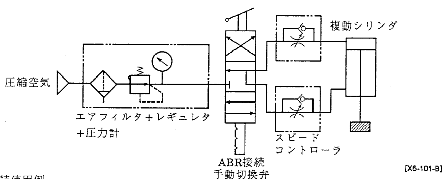
図2. ABR接続使用例
