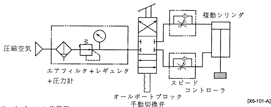
図1. オールポートブロック使用例
