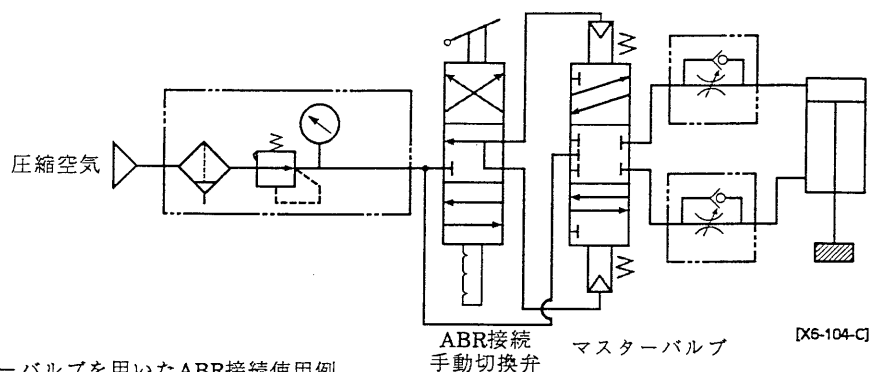
図3. マスターバルブを用いたABR接続使用例
