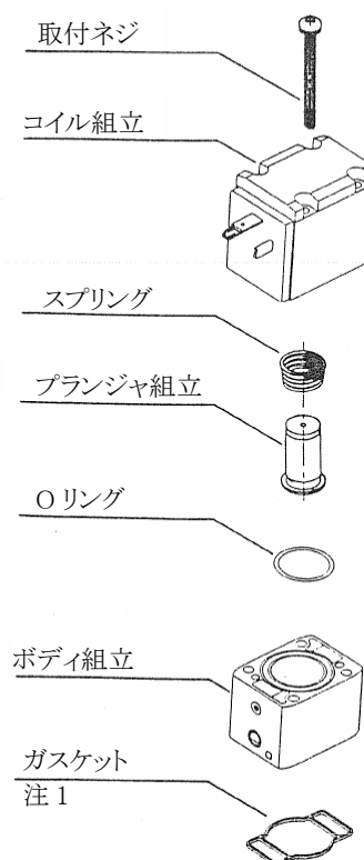
(図 4-4)パイロット用電磁弁の分解図
