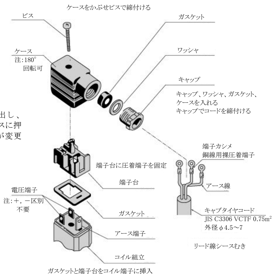
(図 2 - 5) DIN 端子箱の結線方法
