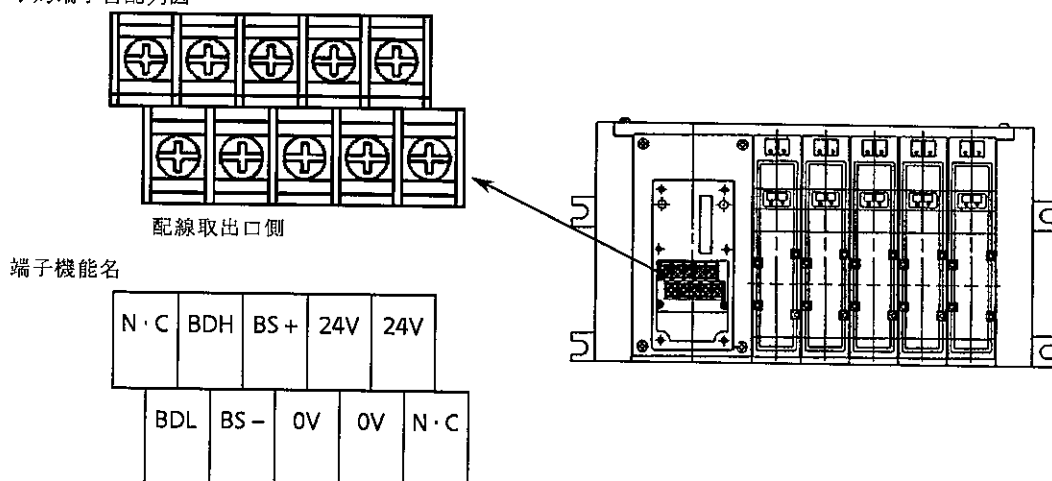
子局端子台配列図
