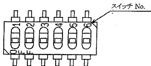
設定用DIPスイッチ
