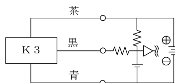
図4 容量性負荷に電流制限抵抗Rを入れた例。 この時の抵抗 R(\Omega) は次式以上を使用してください。
