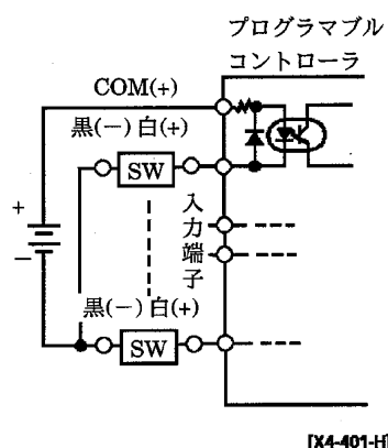
図8 ソース入力 (電源外付) 形へのT2、S2接続例
