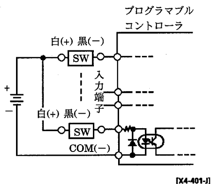
図10 シンク入力形へのT2、S2接続例
