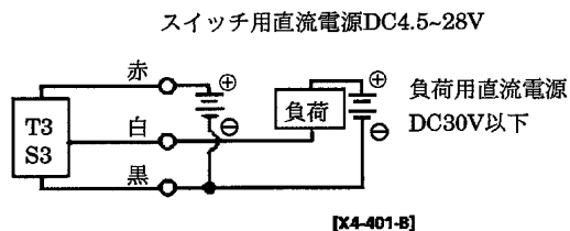
図2 T3、S3基本回路例(2) (スイッチ用電源と負荷用電源が異なる場合)
