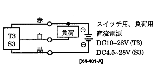
図1 T3、S3基本回路例(1) (スイッチ用電源と負荷用電源が同一の場合)
