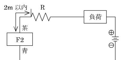
図7・突入電流制限抵抗 R =負荷側回路が許す限り大きな抵抗 ・スイッチの近くで配線する(2m 以内)
