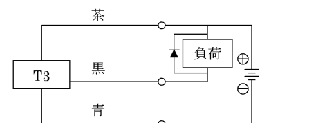
図4 誘導負荷にサージ吸収素子(ダイオード)を使用した例。ダイオードは日立製作所製 V06C、または相当品を使用してください。
