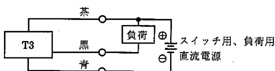
図1 基本回路例(1) (スイッチ電源と負荷用電源が同一の場合)
