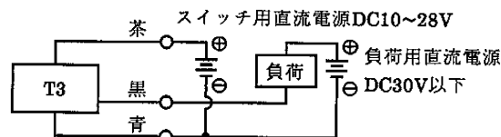
図2 基本回路例(3) (スイッチ電源と負荷用電源が異なる場合)
