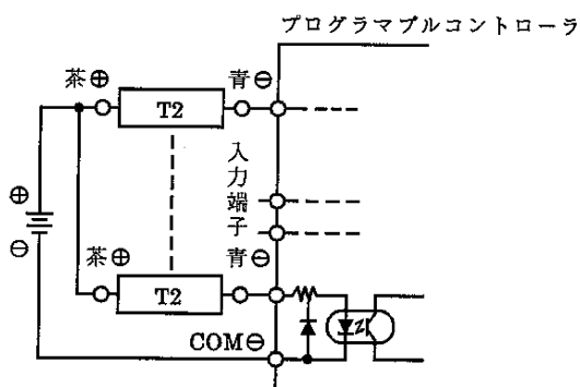
図10 シンク入力形へのT2接続例
