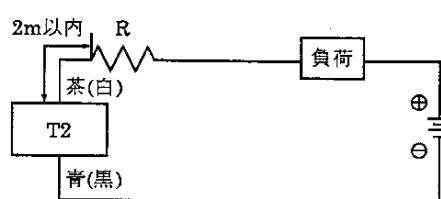
図6 ● 突入電流制限抵抗
