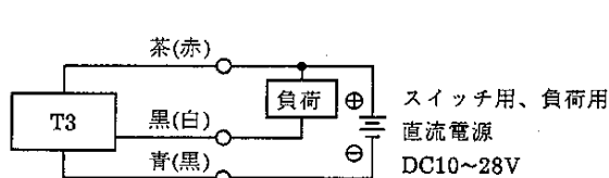
図1 基本回路例(1)(スイッチ電源と負荷用電源が同一の場合)
