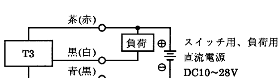
図1 T3基本回路例(1)(スイッチ電源と負荷用電源が同一の場合)
