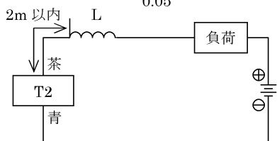
図10・チョークコイル
