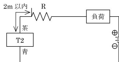
図11・突入電流制限抵抗
