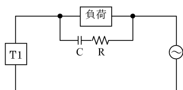
図7:CR回路での保護回路の例
