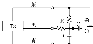
図9 容量性負荷に電流制限抵抗 Rを入れた例。
