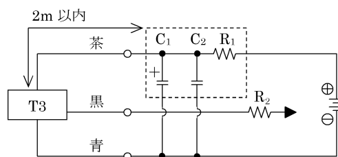
図 10・電源ノイズ吸収回路 C 1 =20~50 μF 電解コンデンサ (耐圧 50V 以上) C 2 =0.01~0.1 μF セラミックコンデンサ R 1 =20~30 Ω ・突入電流制限抵抗 R 2 =負荷側回路が許す限り大きな抵抗を使用 ・スイッチの近くで配線する(2m 以内)
