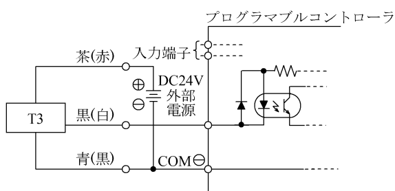
図12 ソース入力(電源内蔵)形へのT3 接続例
