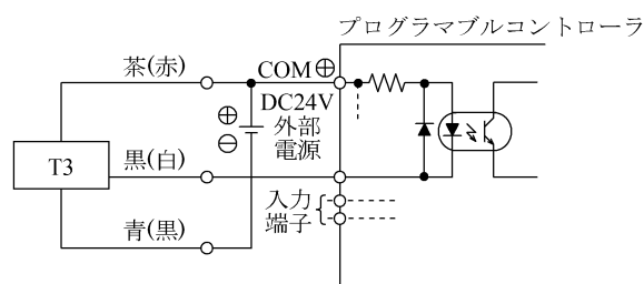
図11 ソース入力(電源外付)形へのT3 接続例
