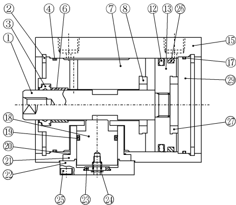
・ SSD-QL-50～100-R (複動・片ロッド形・ロッド側落下防止付)
