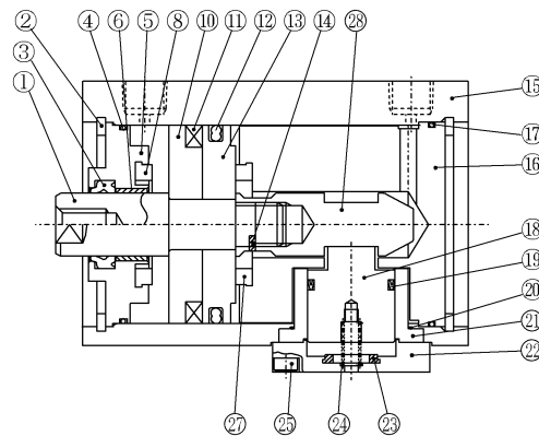
・ SSD-Q-50～100-H (複動・片ロッド形・スイッチ付・ヘッド側落下防止付)
