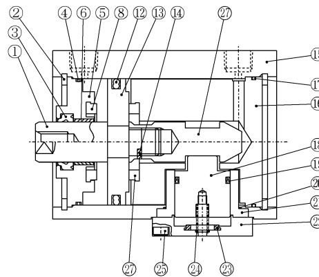
・ SSD-QL-50～100-H (複動・片ロッド形・ヘッド側落下防止付)
