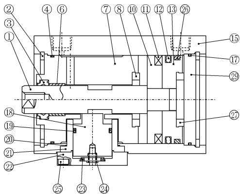
・ SSD-Q-50～100-R (複動・片ロッド形・スイッチ付・ロッド側落下防止付)
