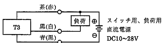
図1 T3基本回路例(1)(スイッチ電源と負荷用電源が同一の場合)
