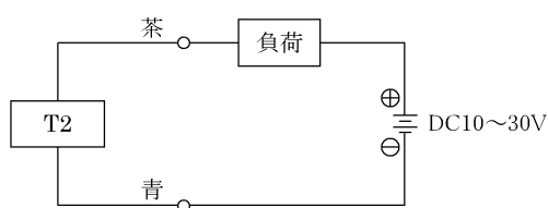
図1 T2 基本回路例
