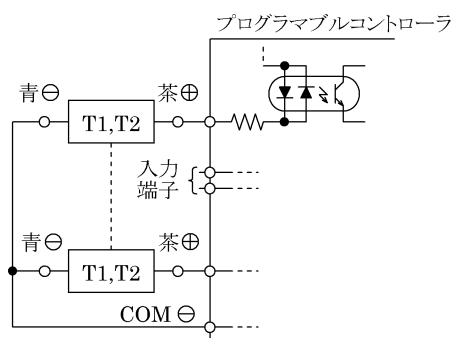
図10 ソース入力(電源内蔵)形への T1,T2 接続例
