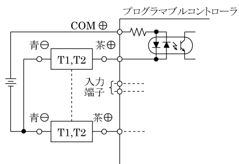
図9 ソース入力(電源外付)形への T1,T2 接続例
