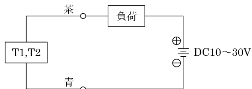
図1 T1, T2 基本回路例
