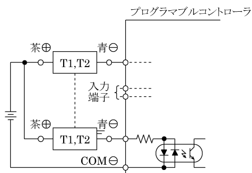
図11 シンク入力(電源外付)形への T1,T2 接続例
