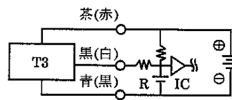
図4 容量性負荷に電流制限抵抗Rを入れた例。この時の抵抗 R(\Omega) は次式以上を使用してください。
