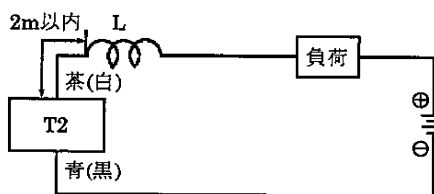
図5 ● チョークコイル
