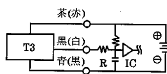
図4 容量性負荷に電流制限抵抗Rを入れた例。この時の抵抗 R(\Omega) は次式以上を使用してください。
