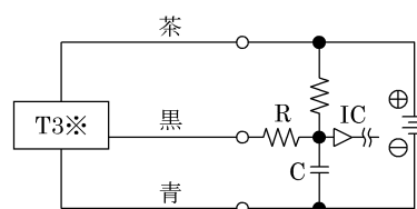
図4 容量性負荷に電流制限抵抗 R を入れた例。 この時の抵抗は次式の R(Ω) 以上を使用してください。
