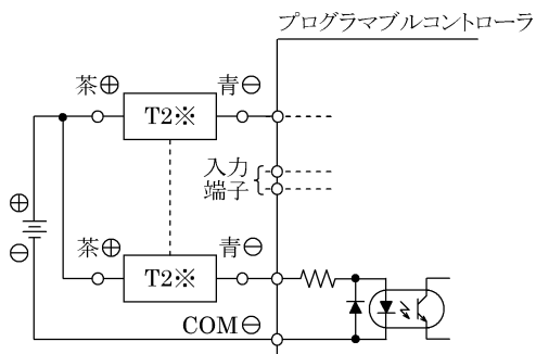
図10 シンク入力(電源外付)形へのT2※接続例
