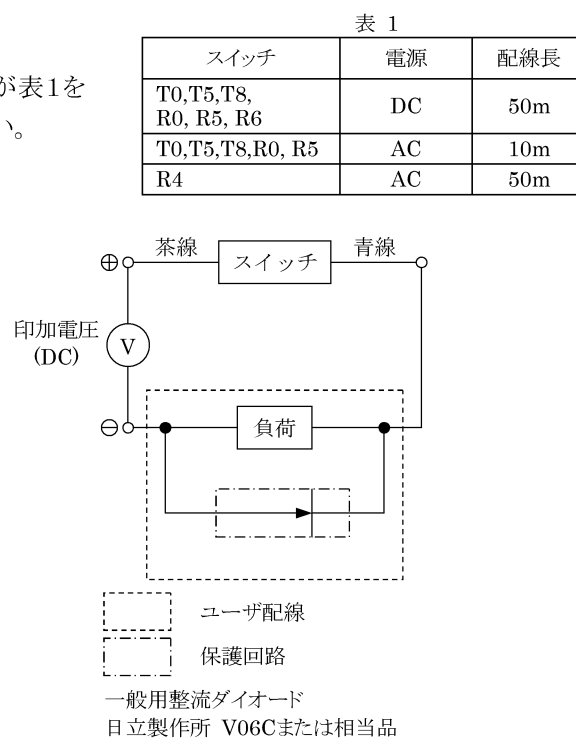
図2 ダイオード使用時
