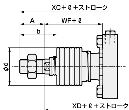
〈ジャバラ付〉
