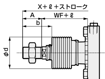
〈ジャバラ付〉
