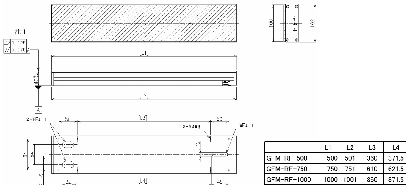
GFM-RF-＊ 外形図
