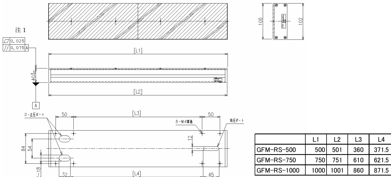
GFM-RS-＊ 外形図
