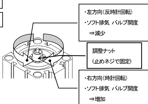
調整ナット拡大図
