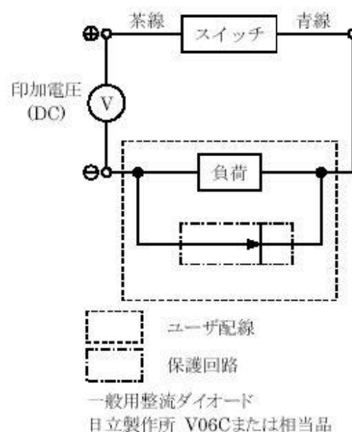
図2 ダイオード使用時
