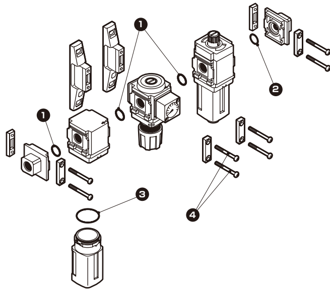
■C1000-W 部品展開図
