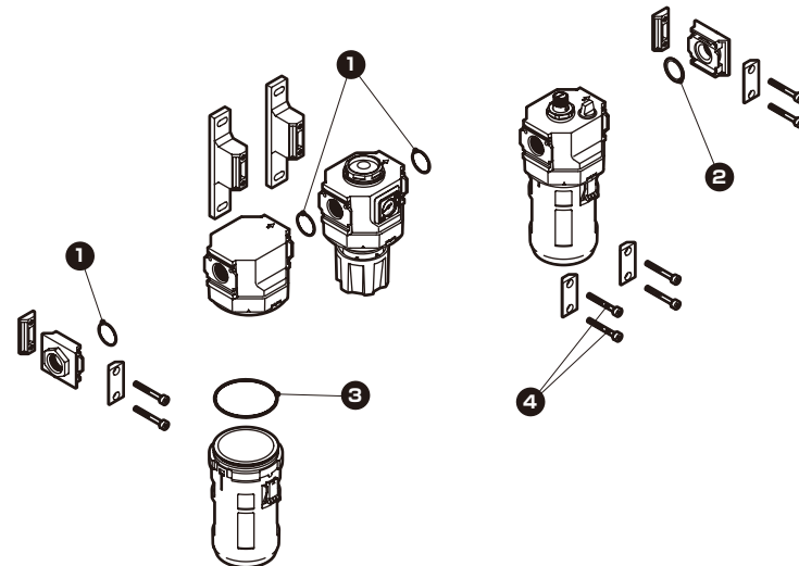
■C2000/2500/3000/4000-W 部品展開図
