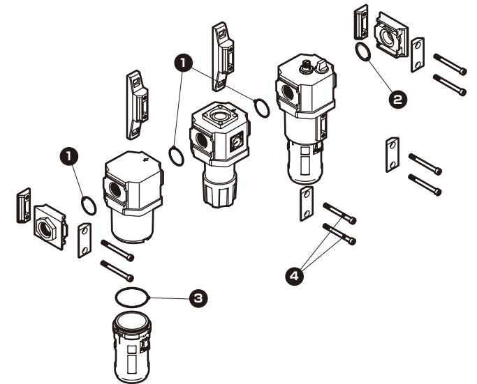
■C6500/8000-W 部品展開図
