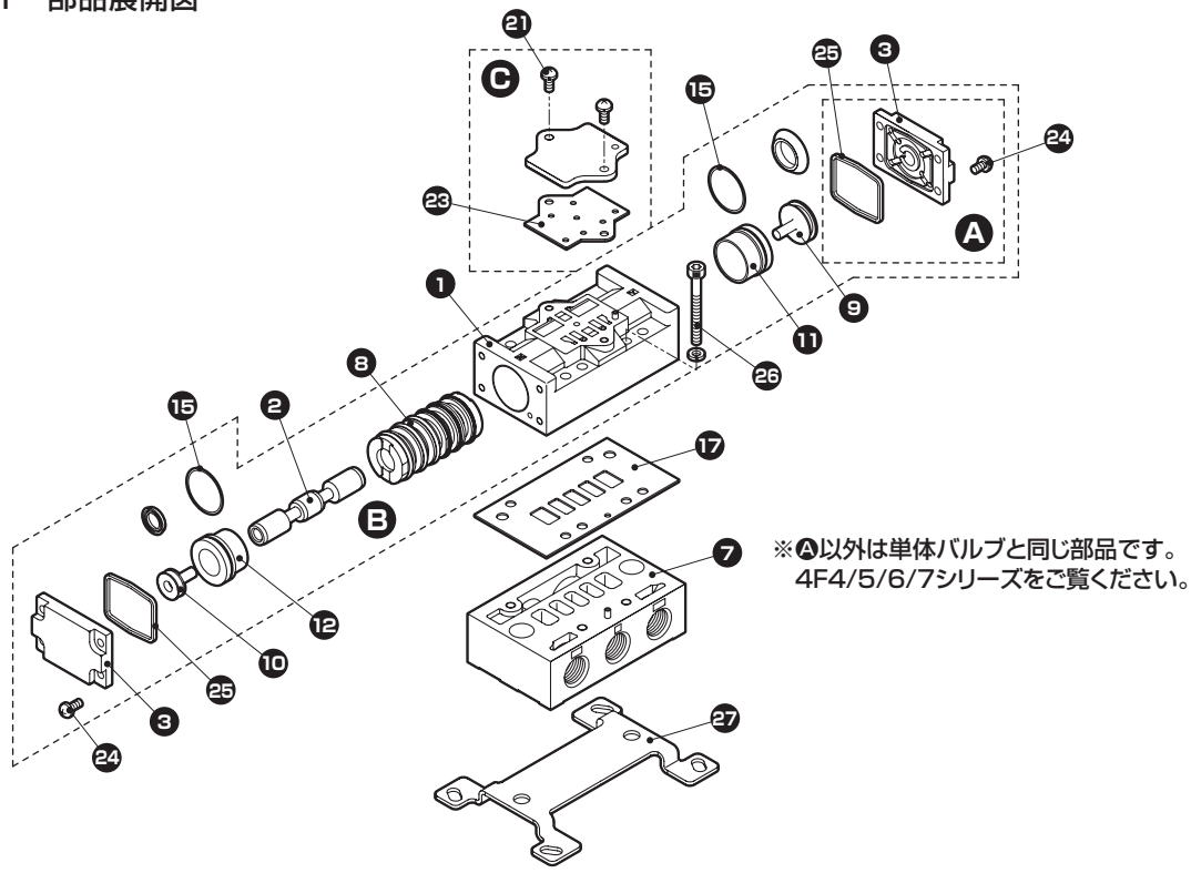
●4F4 4 / 5 11 部品展開図
