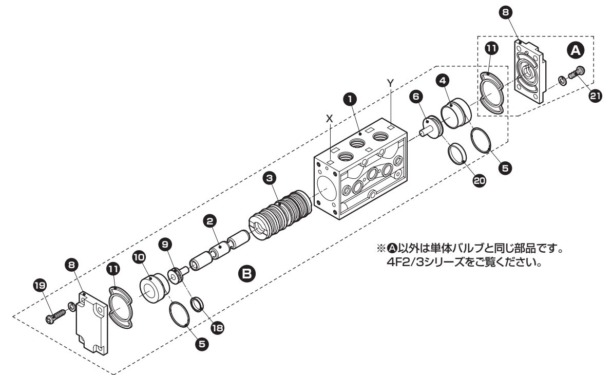
●4F 3 2 11 部品展開図
