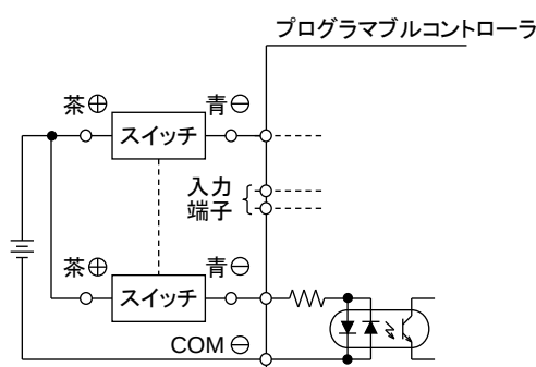
シンク入力(電源外付)形への2線式接続例
