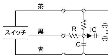
例 2 容量性負荷に電流制限抵抗 R を入れた例。 この時抵抗 R(Ω)は次式以上を使用してください。
