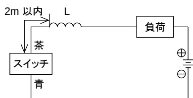
例 3 ・チョークコイル L=数百 \mu\text{H} ~ 数 mH 高周波特性にすぐれたもの ・スイッチの近くで配線する(2m 以内)
