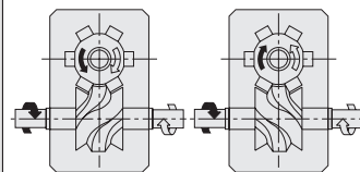
左ねじれ (標準)
