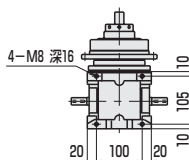
B 矢視
