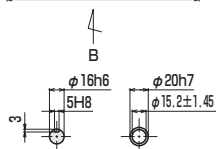
入力軸 固定軸中空穴径
