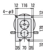
A 矢視
