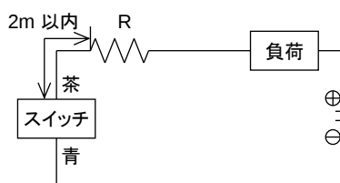
例 4 ・ 突入電流制限抵抗 R=負荷側回路が許すかぎり大きな抵抗 ・ スwitchの近くで配線する(2m 以内)
