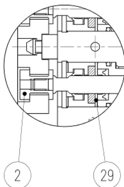
A 部φ8の場合
