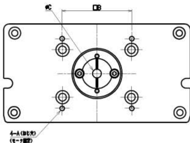
【ECS-14-※※※※※-E】（モータサイズ:C &lt;□60&gt;）
