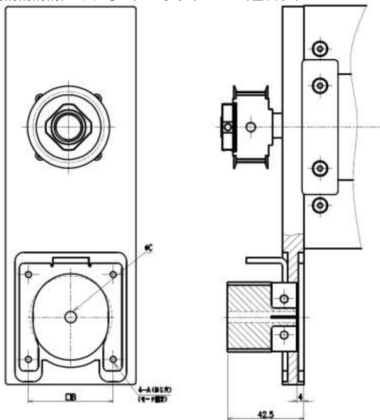
【ECS-14※※※※※- R/L/D】 (モータサイズ:C &lt;□60&gt;)
