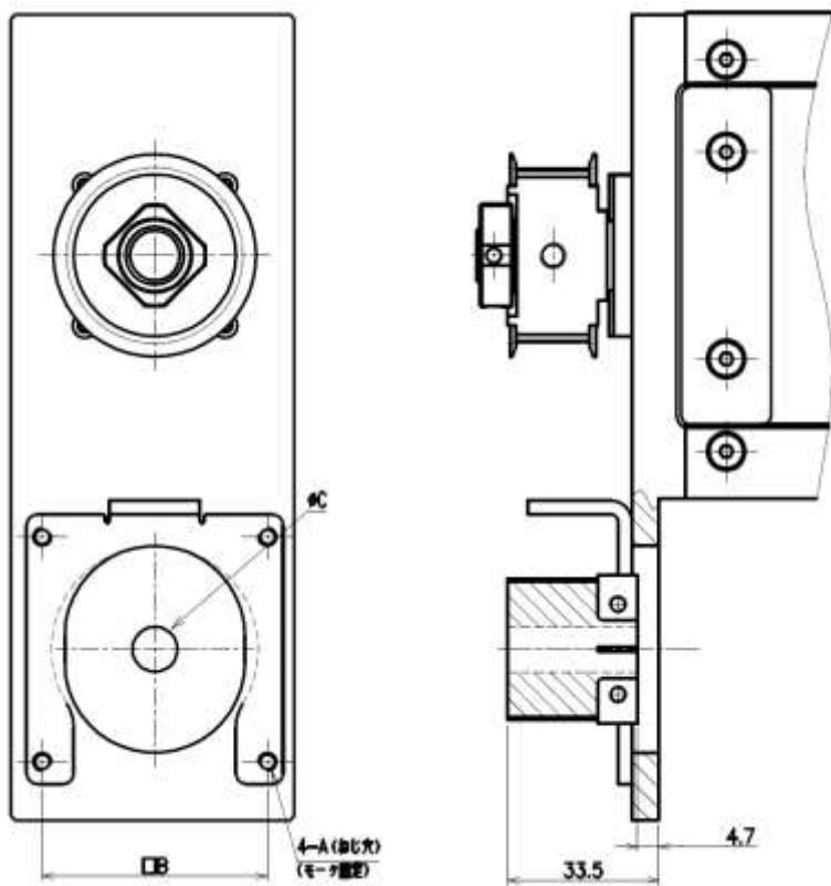
【ECS-12-※※※※※- R/L/D】 (モータサイズ:C &lt;□60&gt;)
