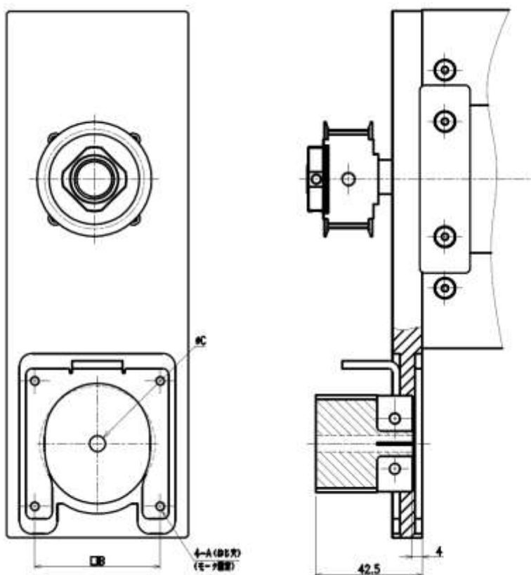
【ECS-14※※※※※- R/L/D】 (モータサイズ:C &lt;□60&gt;)
