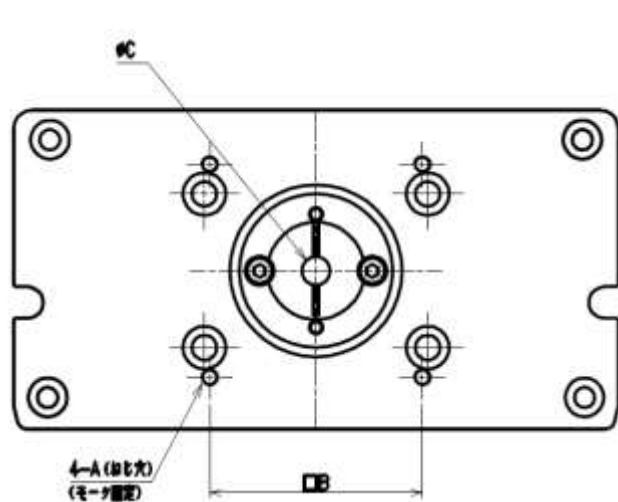
【ECS-14-※※※※※-E】（モータサイズ:B &lt;□56&gt;）
