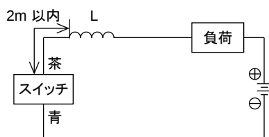
例 3 ・ チョークコイル L=数百 \mu\text{H} ~ 数 \text{mH} 高周波特性にすぐれたもの ・ スwitch の近くで配線する(2m 以内)
