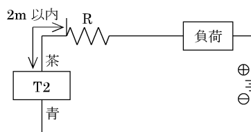
図7 起動電流制限抵抗 R = \text{負荷側回路が許す限り大きな抵抗} ・スイッチの近くで配線する(2m 以内)
