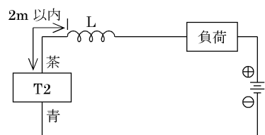
図6・チョークコイル L = \text{数百} \mu\text{H} \sim \text{数 mH} 高周波特性にすぐれたもの ・スイッチの近くで配線する(2m 以内)
