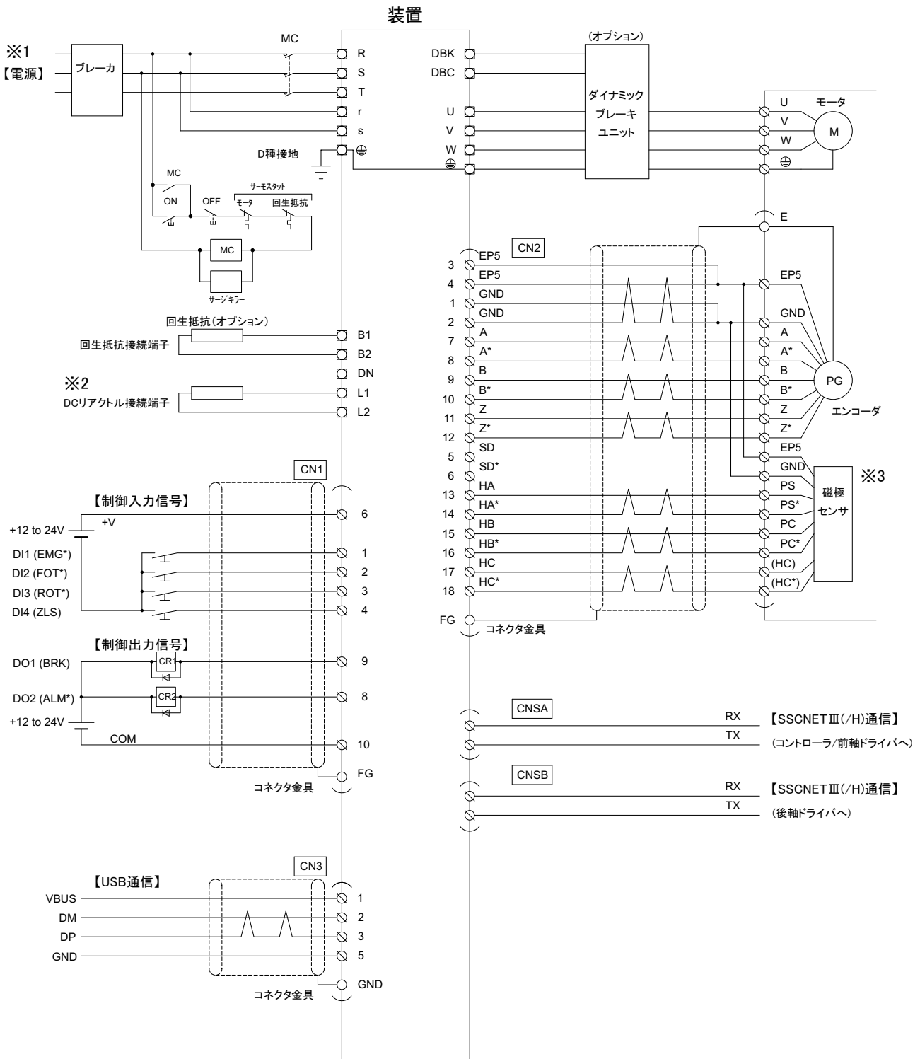
図3-1 外部接続図
