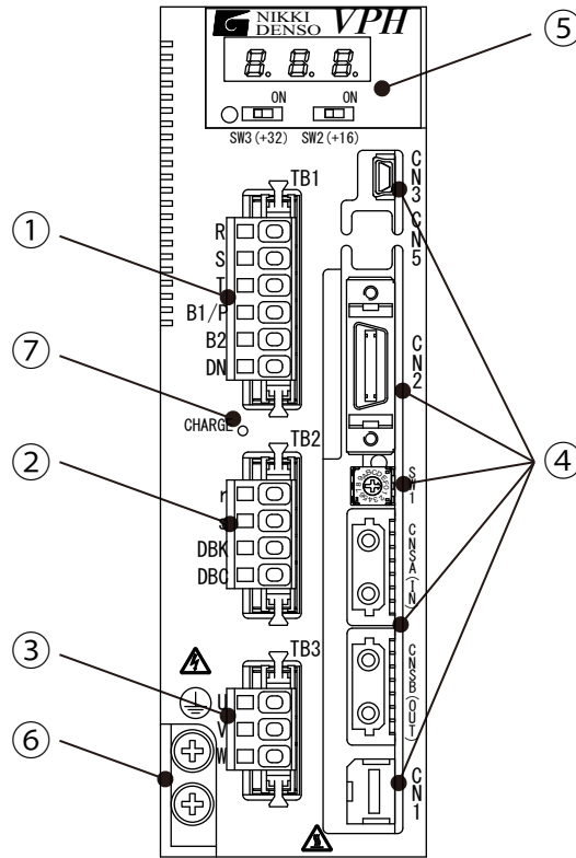
図12-2 400W以下装置本体正面図 (Type1)
