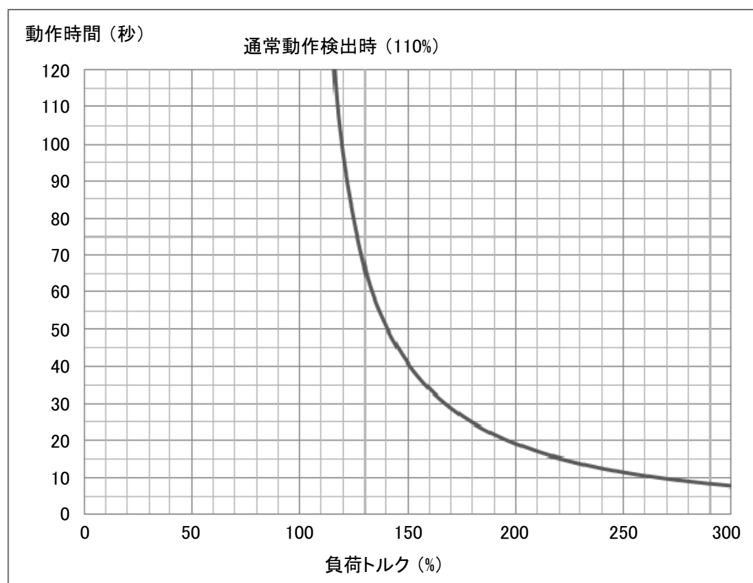
図8-1 負荷トルクと検出時間の関係
