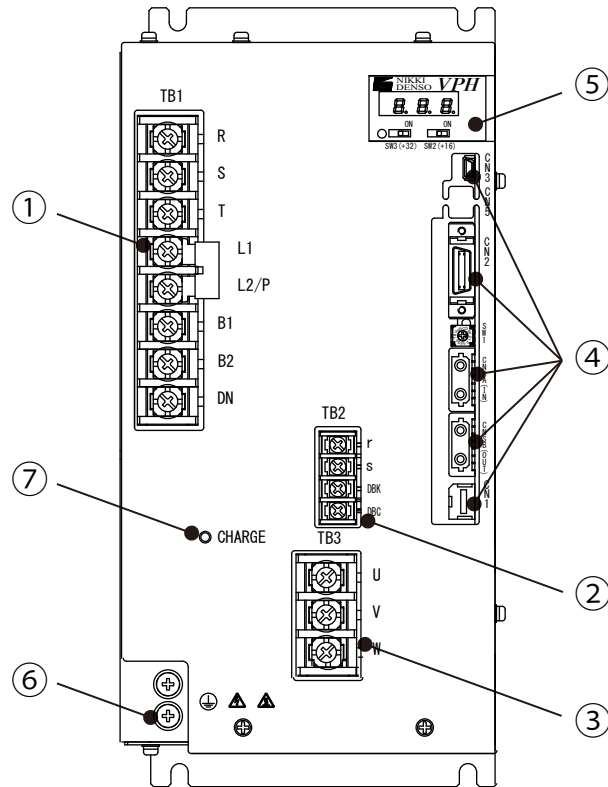
図12-8 3.3kW装置本体正面図 (Type4)
