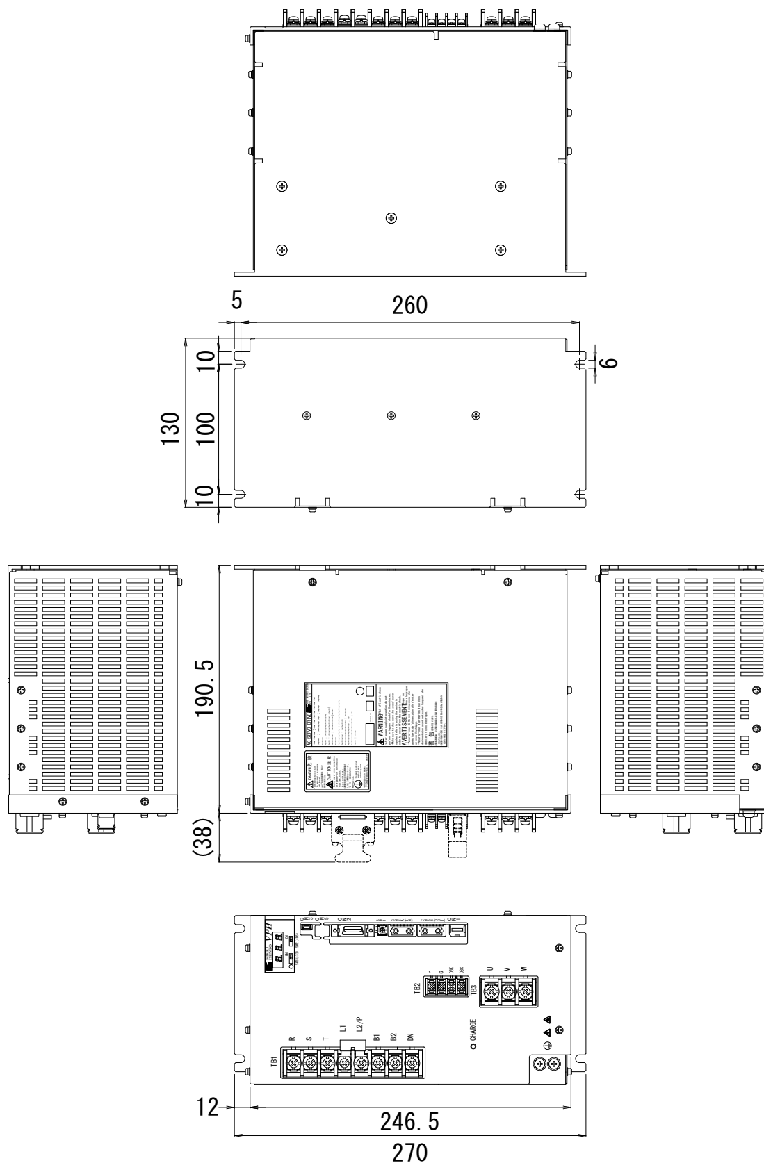
図12-7 3.3kW装置本体外形図(Type4)
