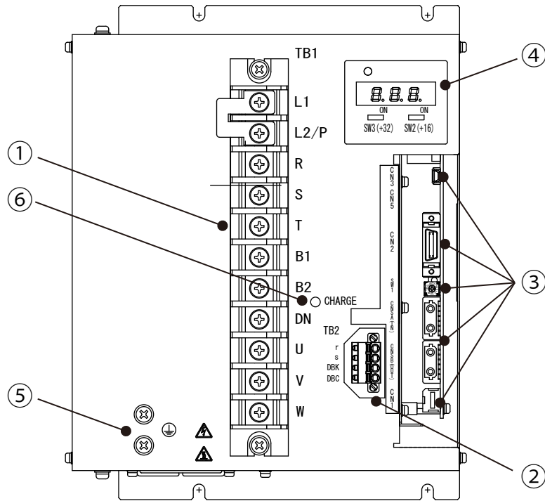
図12-10 7kW装置本体正面図 (Type5)
