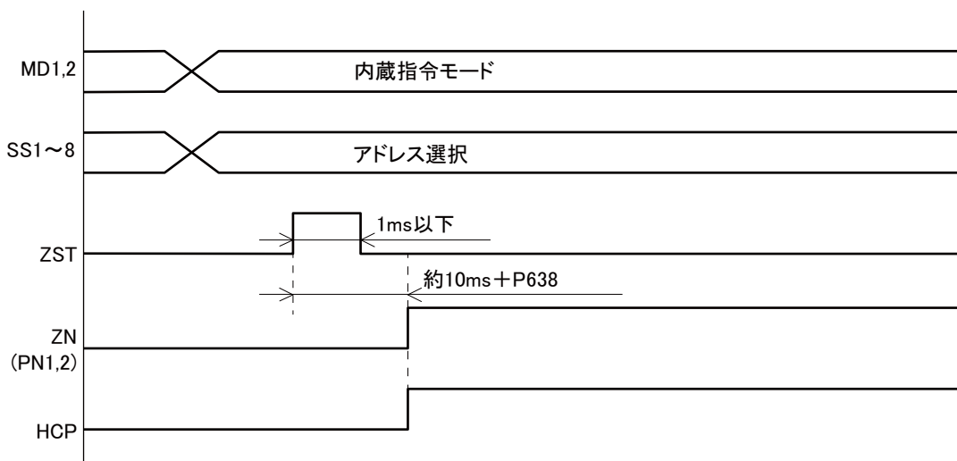
図5-17 SET ABS タイムチャート
