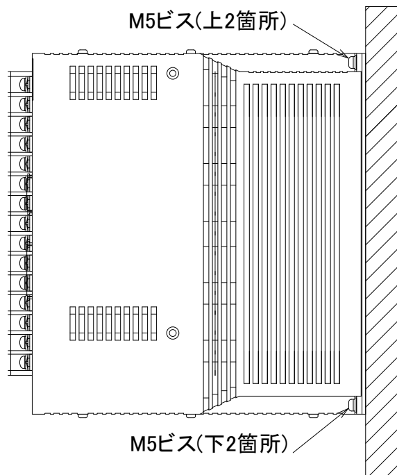
図2-4 装置の取付け方法(1.5kW、2.2kW)
