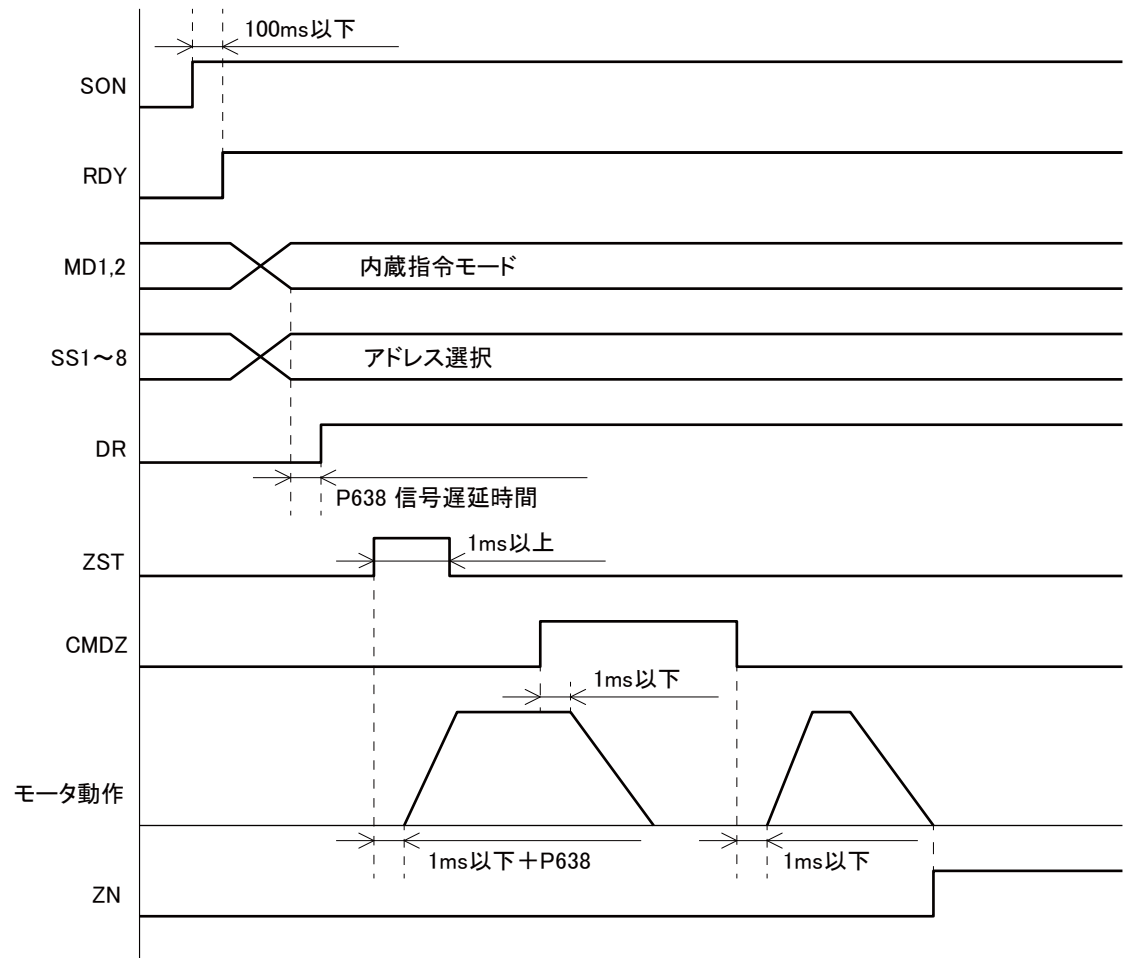
図5-20 INDXコマンドタイムチャート
