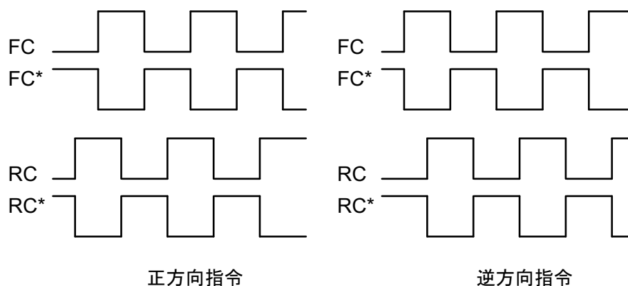
図3-3 90° 位相差信号
