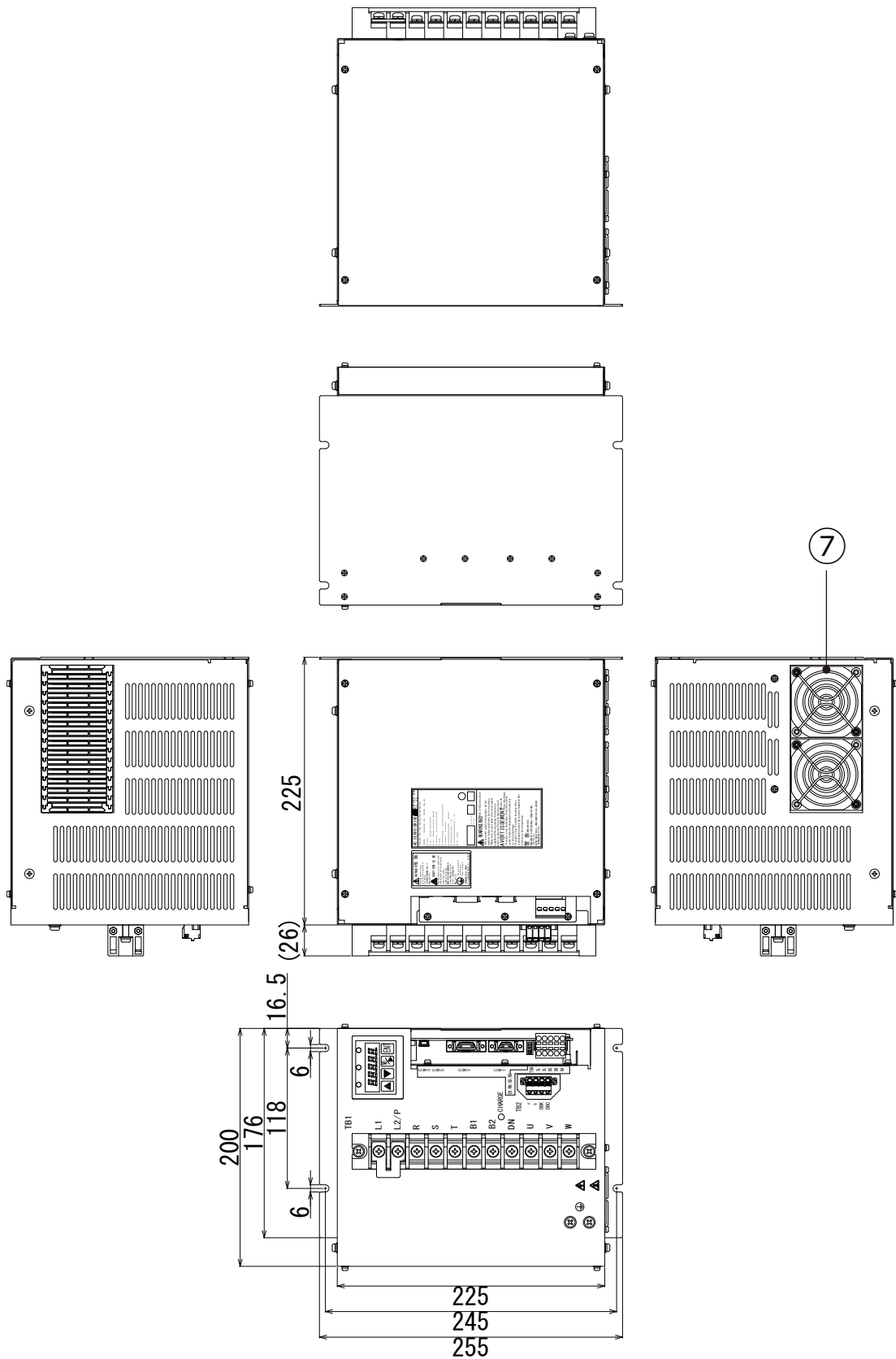
图13-9 7kW装置本体外形图(Type5)
