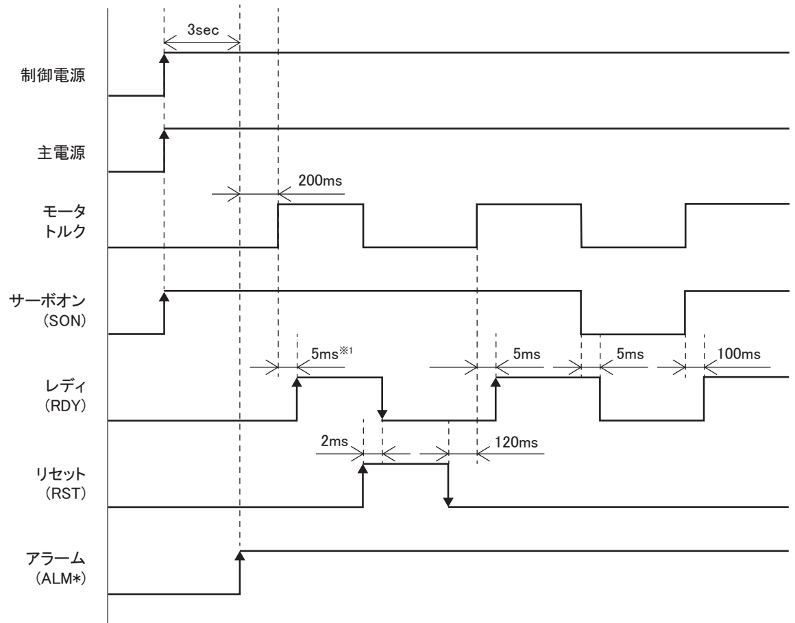
図2-8 タイミングチャート
