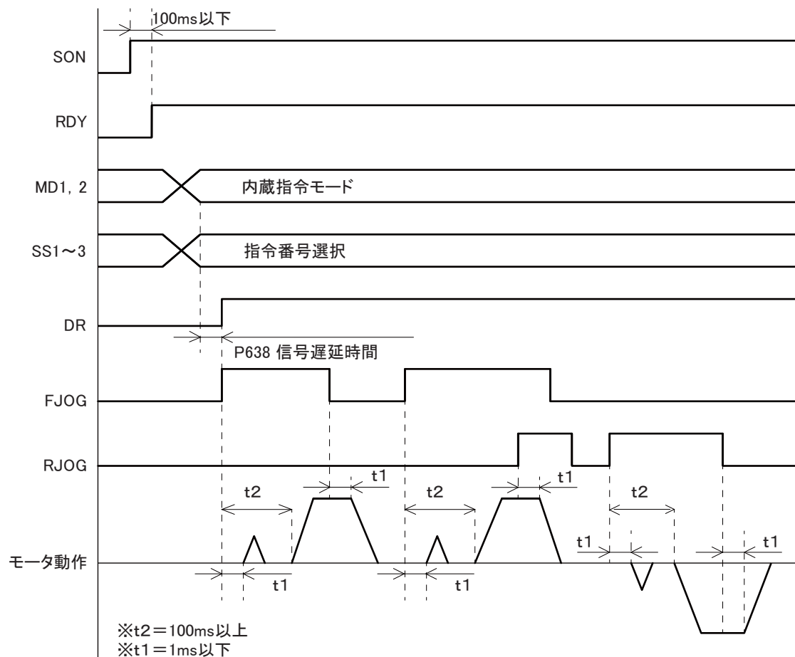
図5-7 寸動動作タイムチャート
