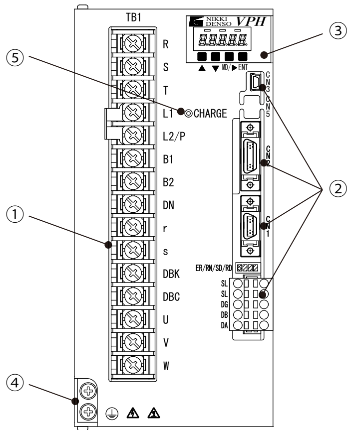
図13-6 1.5kW、2.2kW装置本体正面図 (Type3)
