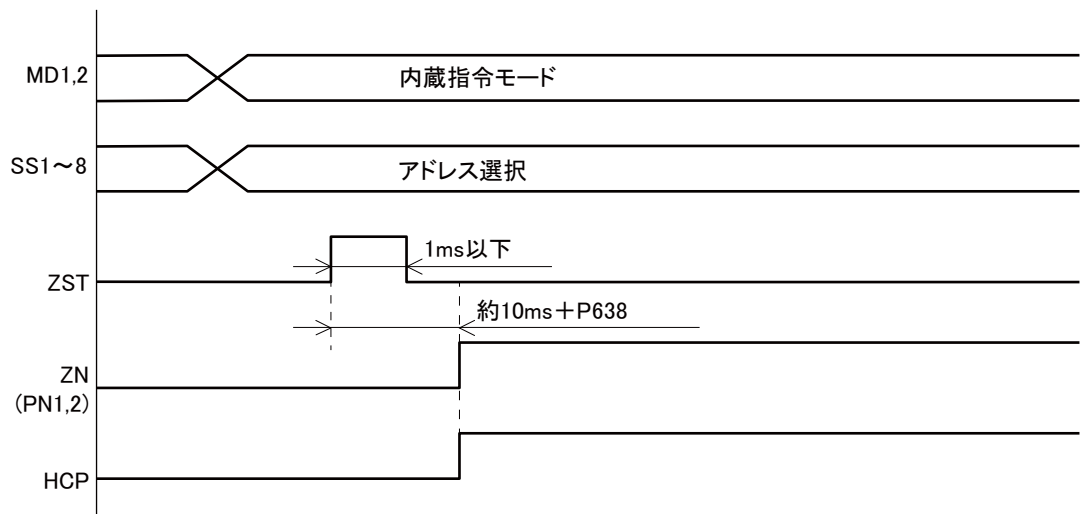
図5-19 SET ABS タイムチャート
