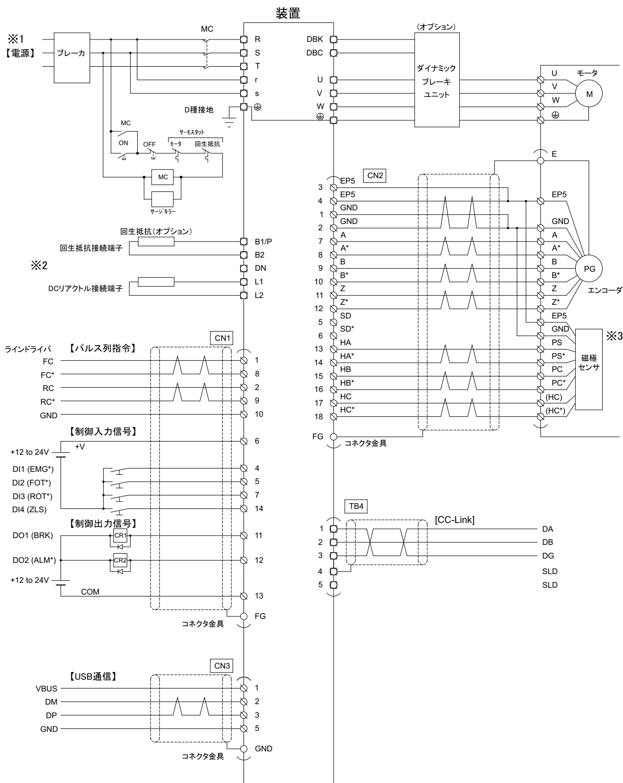
図3-1 外部接続図
