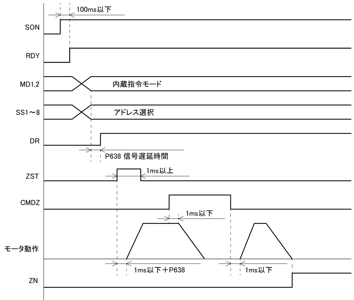
図5-10 POSコマンドタイムチャート
