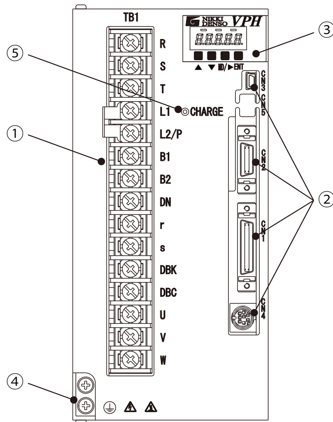
図13-6 1.5kW、2.2kW装置本体正面図 (Type3)
