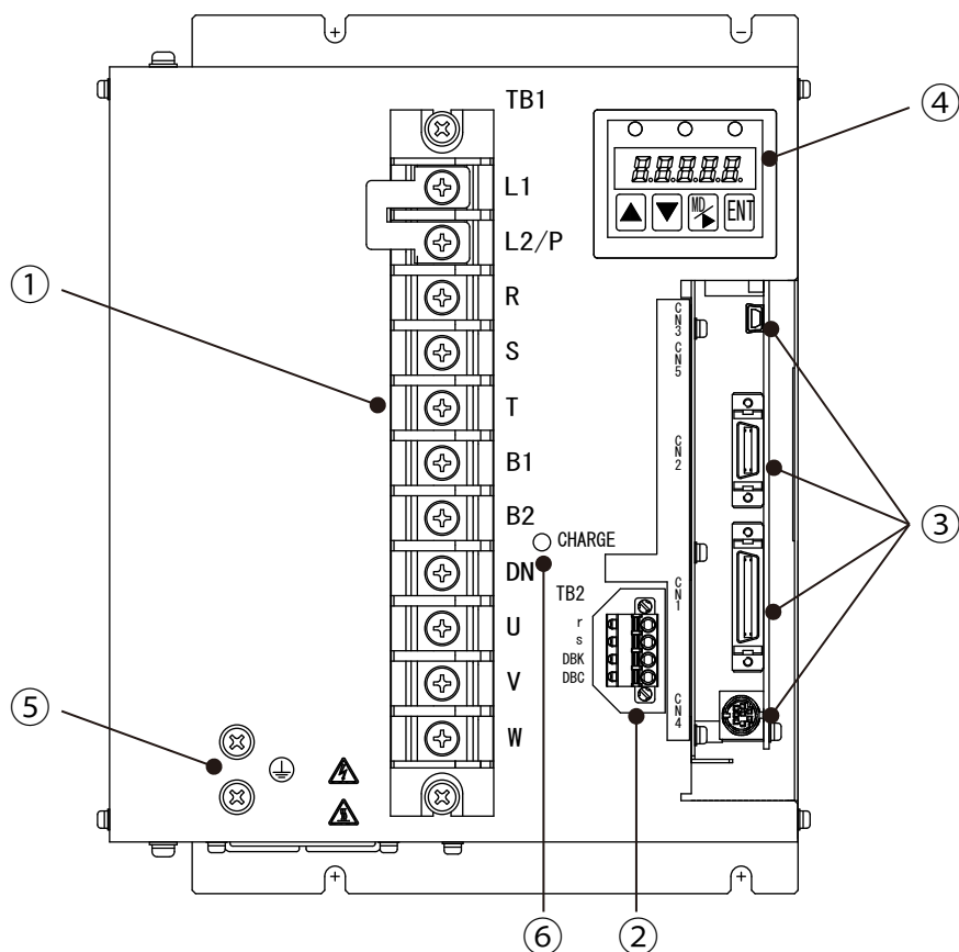
図13-10 7kW装置本体正面図 (Type5)
