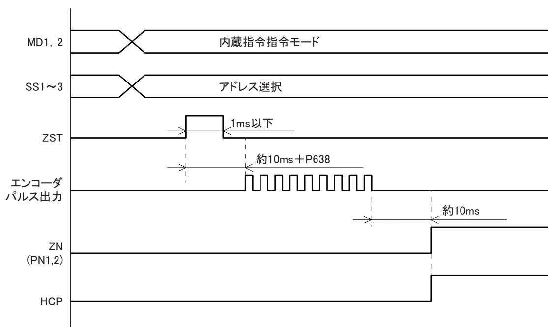
図5-28 OUT POS タイムチャート
