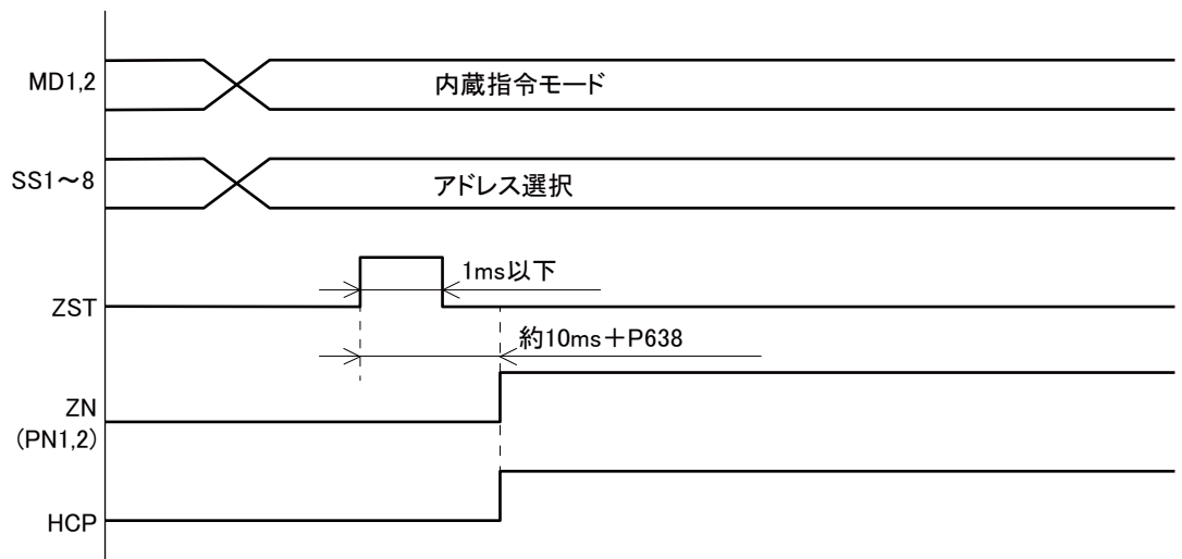
図5-27 SET ABS タイムチャート
