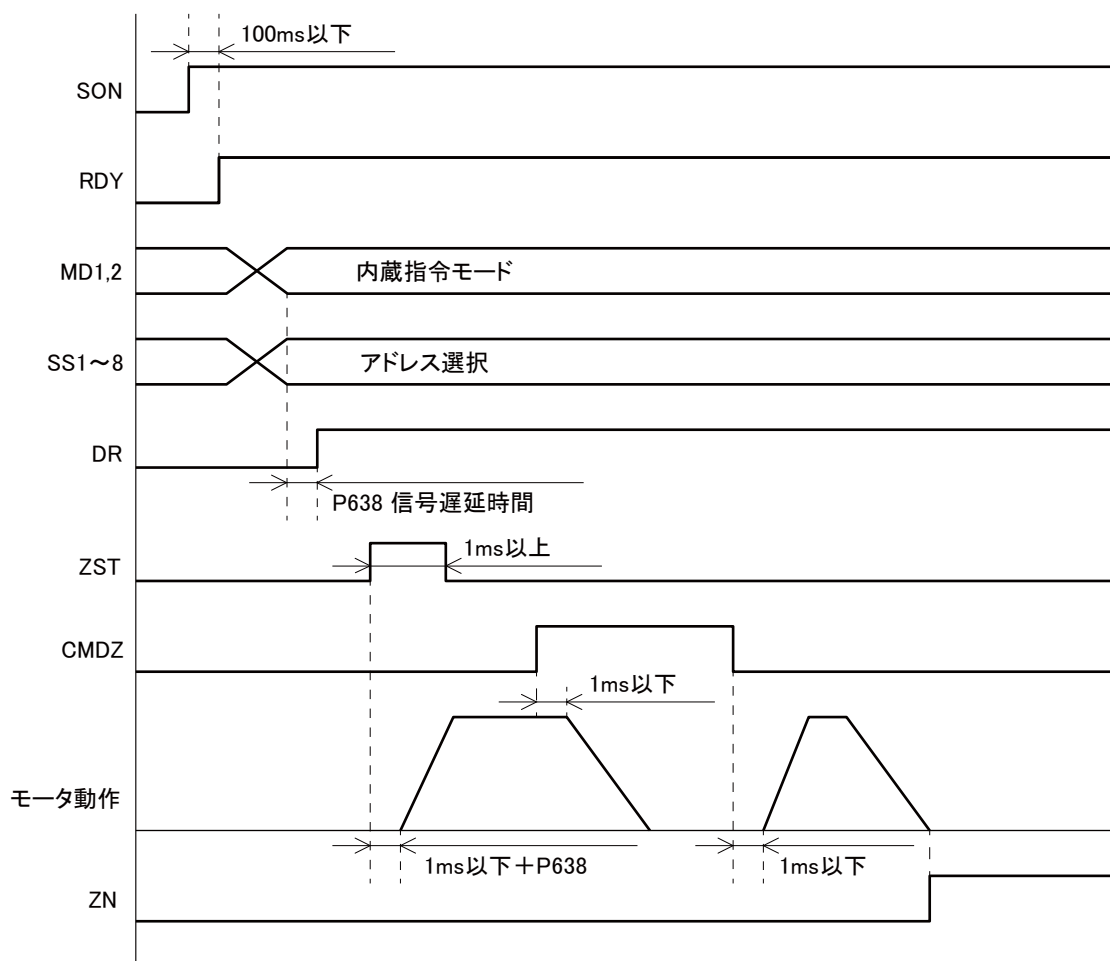
図5-29 INDXコマンドタイムチャート
