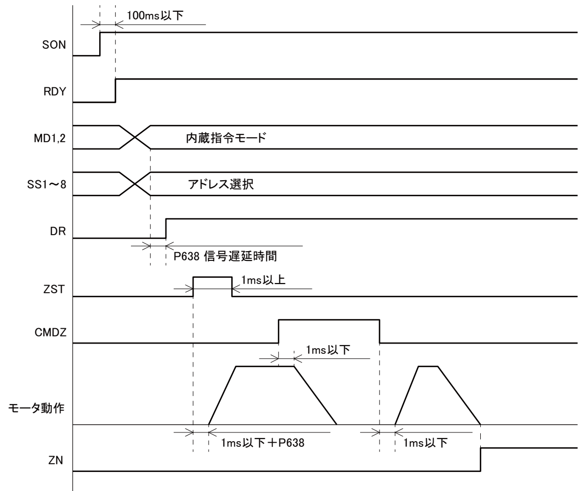
図5-18 POSコマンドタイムチャート
