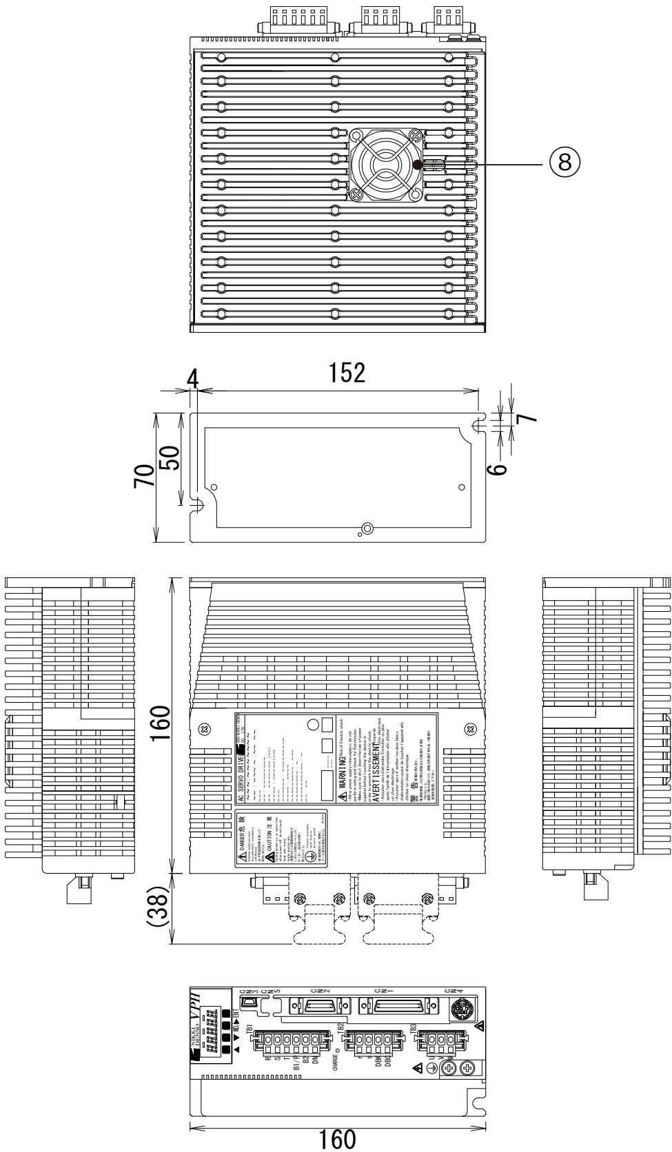
図13-3 800W装置本体外形図(Type2)
