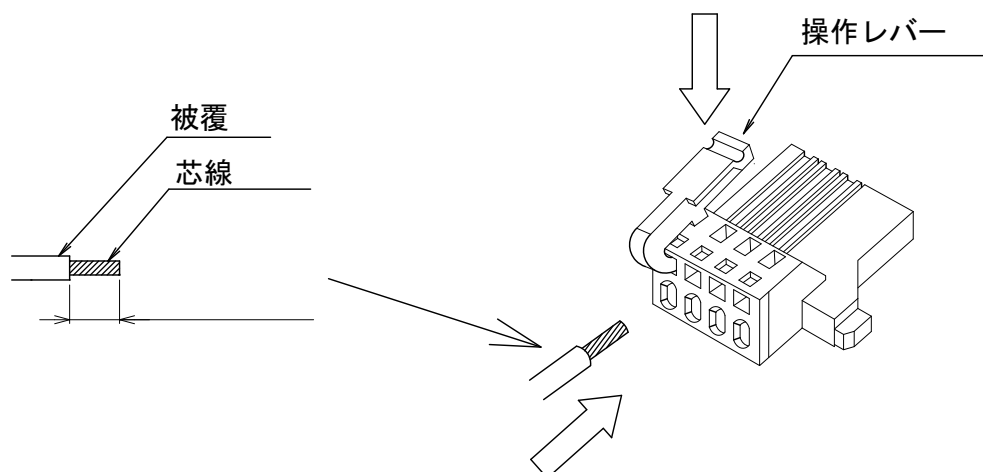
図2-11 プラグコネクタ配線図
