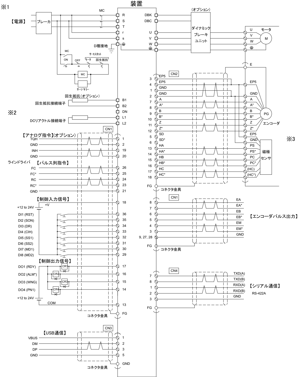
図3-1 外部接続図
