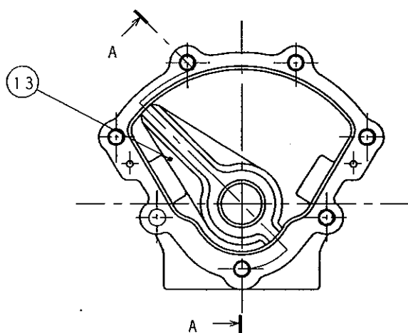
アクチュエータ部内部構造図
