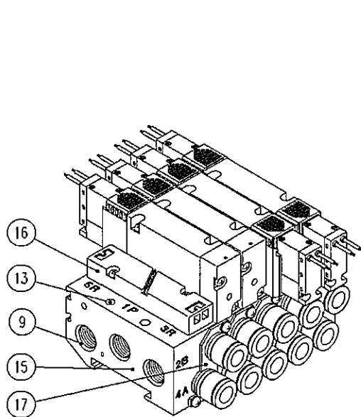
個別配線マニホールド
