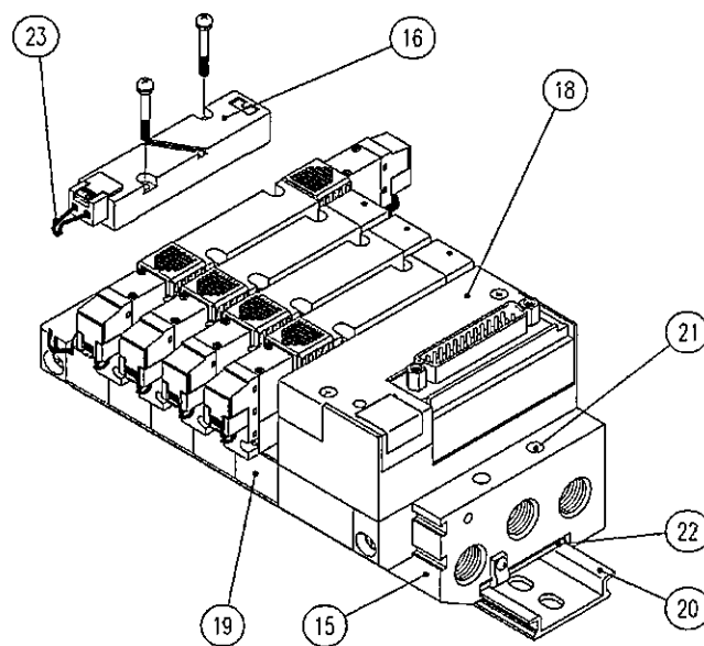
省配線マニホールド(図はDINレール付)
