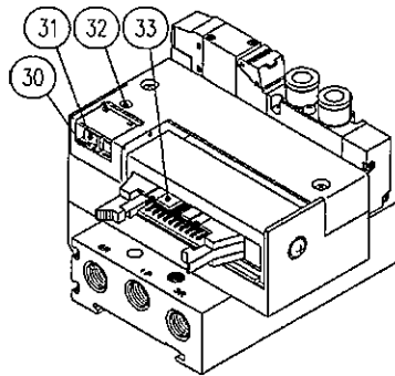
フラットケーブルコネクタ(T50)
