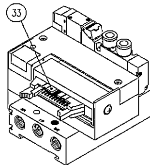
フラットケーブルコネクタ(T51)
