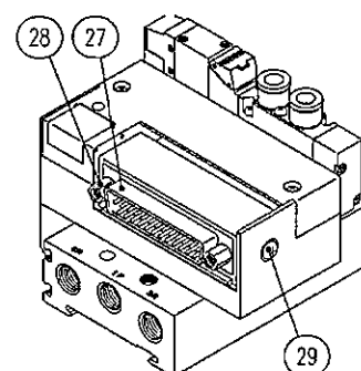
Dサブコネクタ(T30)
