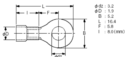
丸形圧着端子外形寸法
