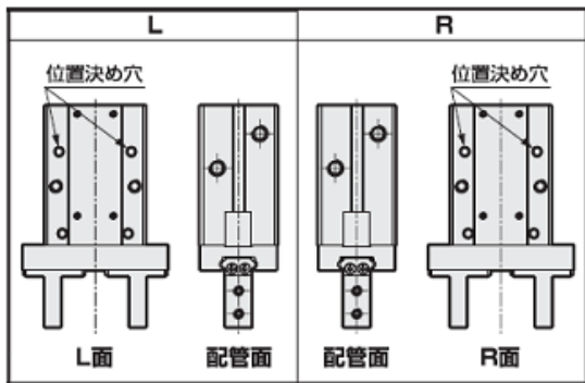
把持センター基準、 高精度位置決め穴位置図
