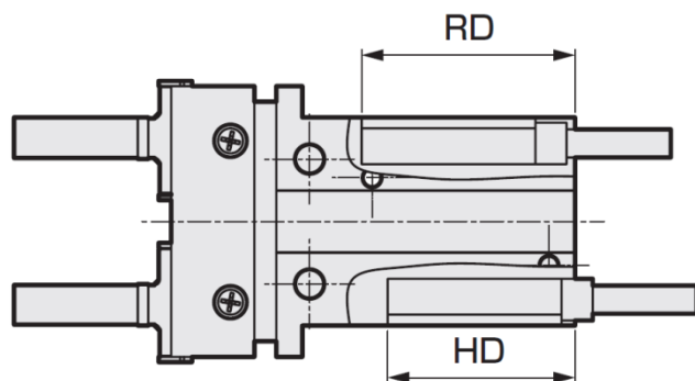
スイッチ付 側面組付
