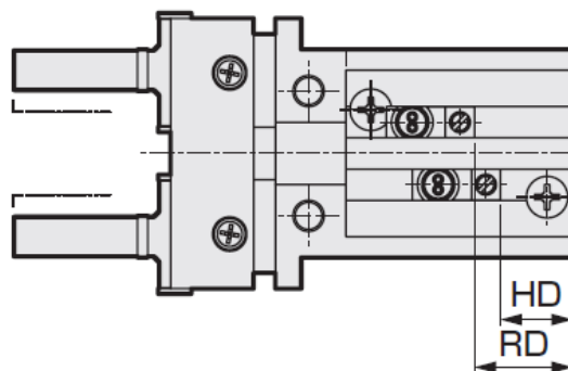
スイッチ付 レール組付
