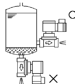
(図2) タンクからの排水回路
