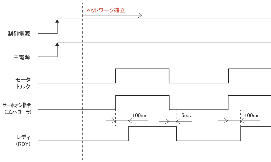
図2-11 タイミングチャート
