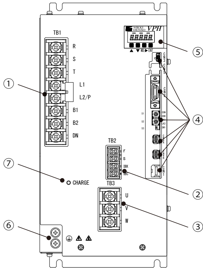
図13-8 3.3kW装置本体正面図 (Type4)
