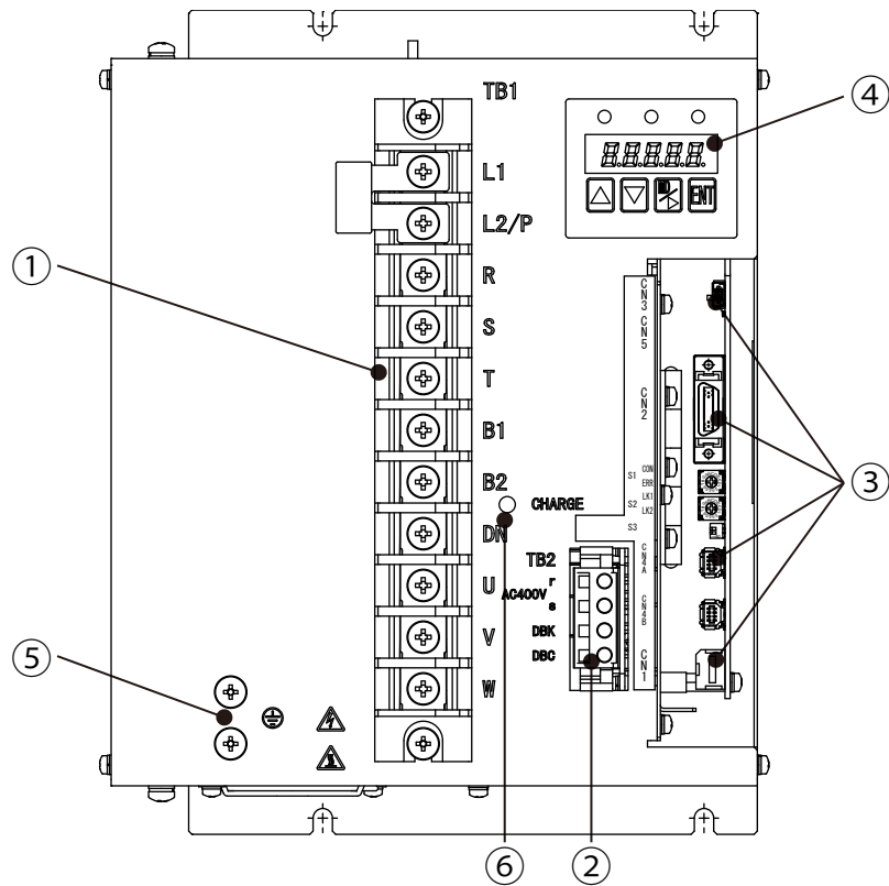
図13-14 400V 7kW装置本体正面図 (Type7)
