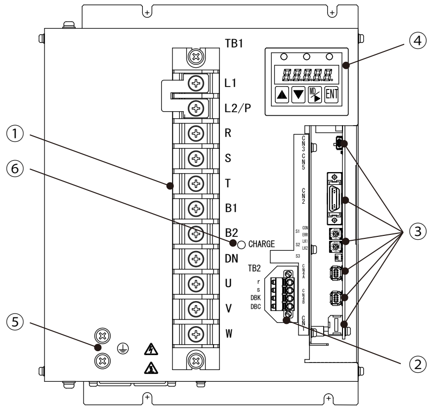
図13-10 200V 7kW装置本体正面図 (Type5)
