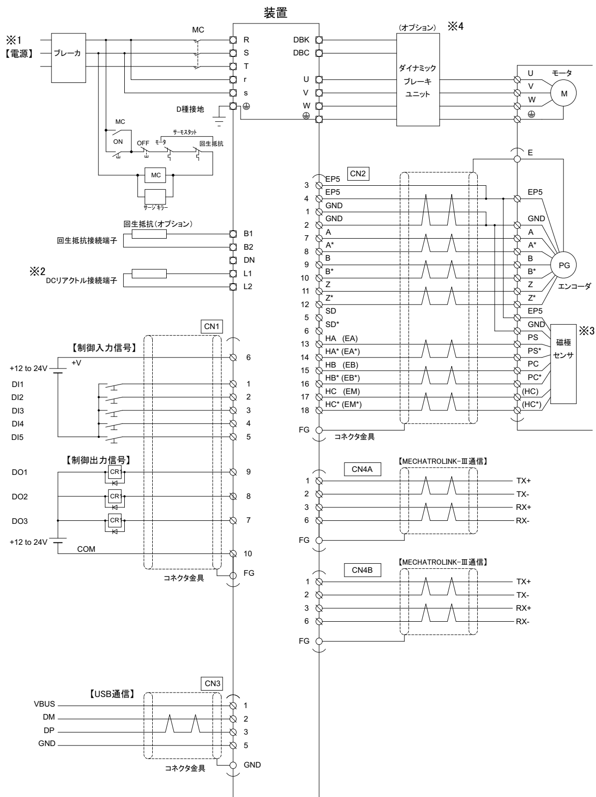
図3-1 外部接続図
