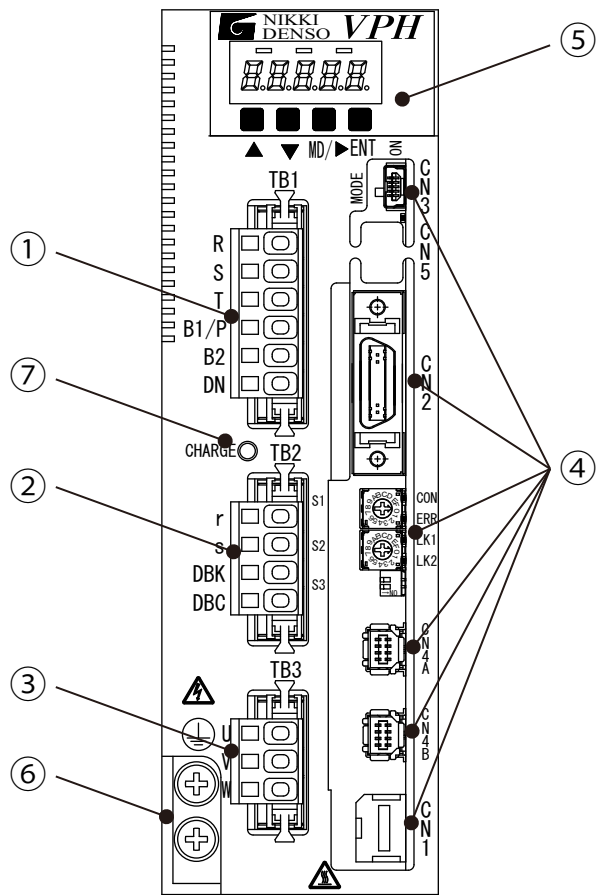
図13-2 400W以下装置本体正面図 (Type1)
