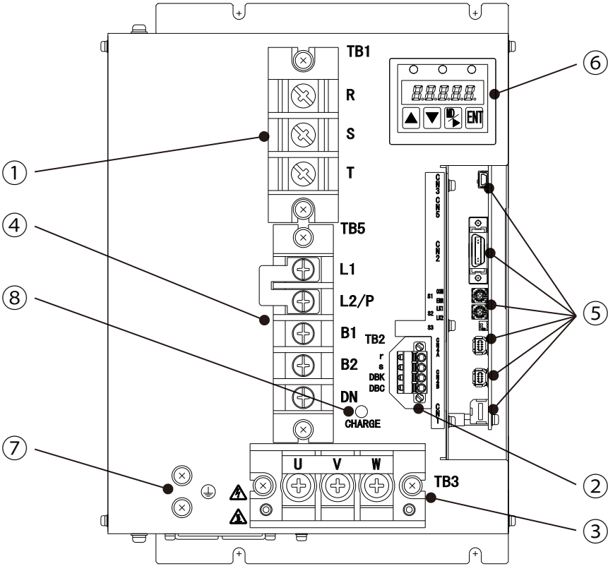
図13-12 15kW装置本体正面図(Type6)
