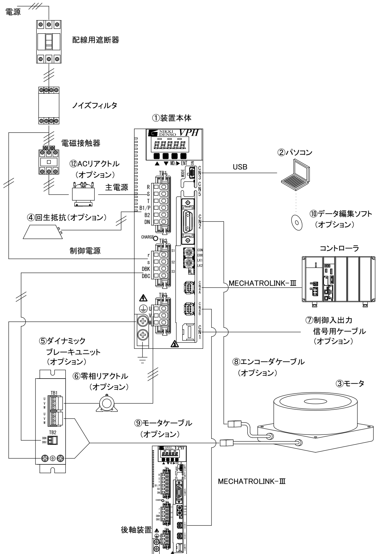
図1-1 800Wクラス以下VPH HEタイプ システム構成
