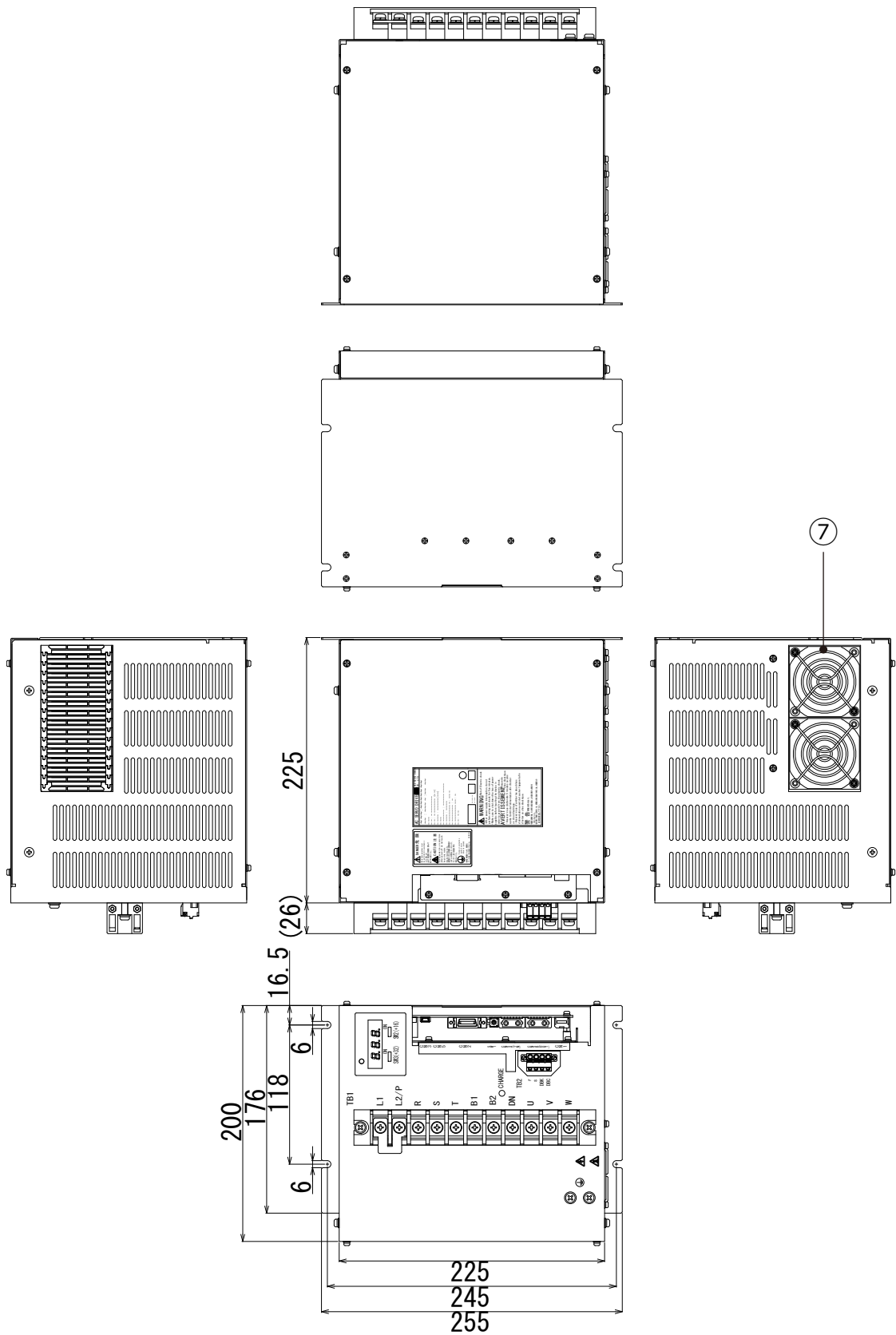
図12-9 200V 7kW装置本体外形図 (Type5)
