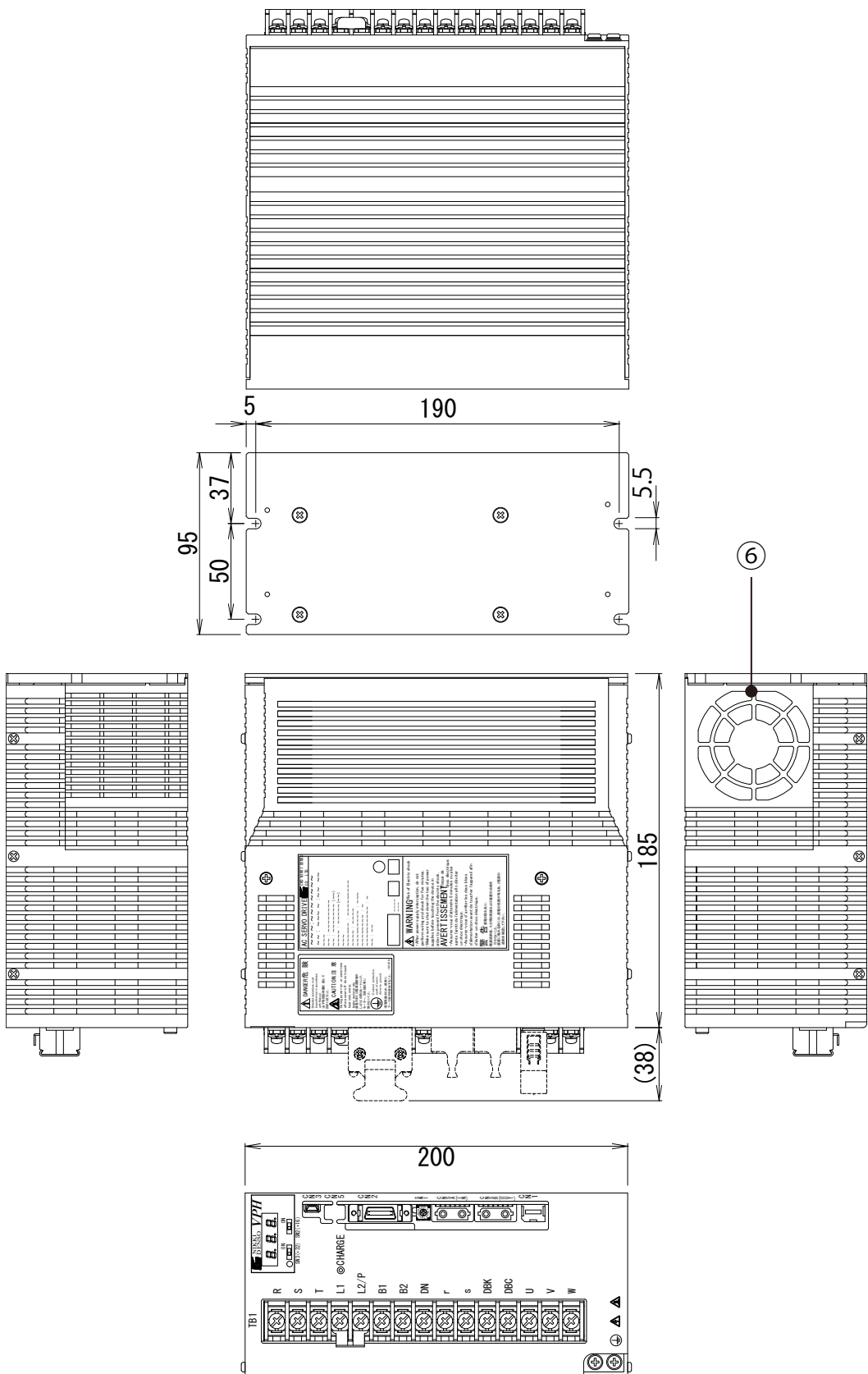
図12-5 1.5kW、2.2kW装置本体外形図 (Type3)
