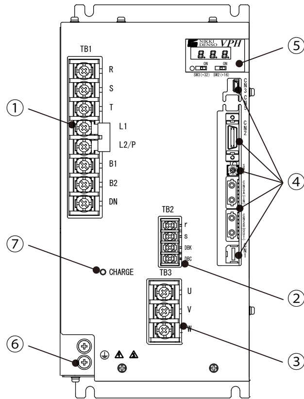
図12-8 3.3kW装置本体正面図 (Type4)
