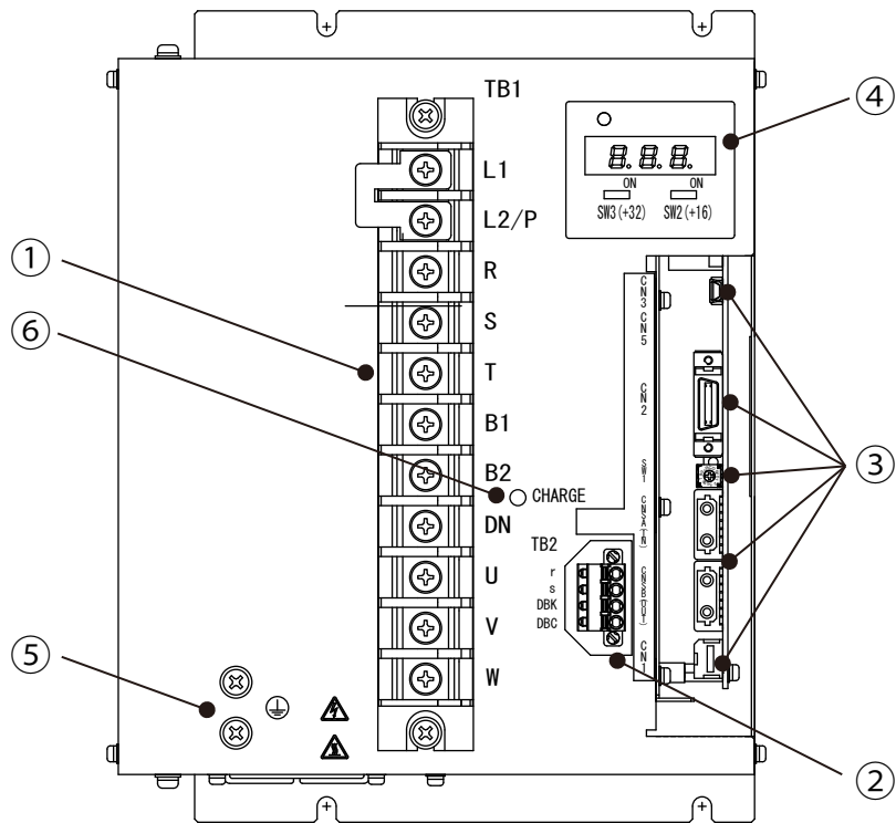
図12-10 200V 7kW装置本体正面図 (Type5)
