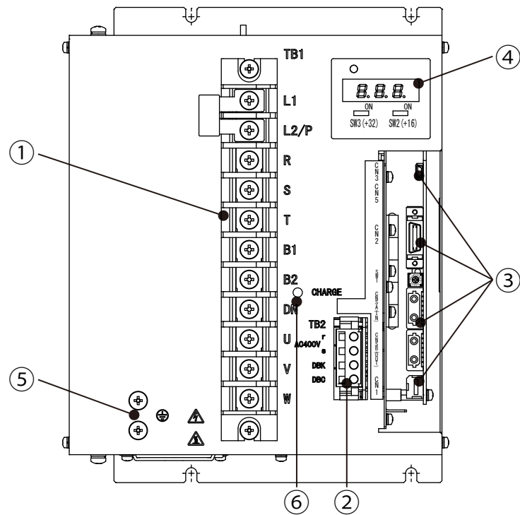
図12-14 400V 7kW装置本体正面図 (Type7)
