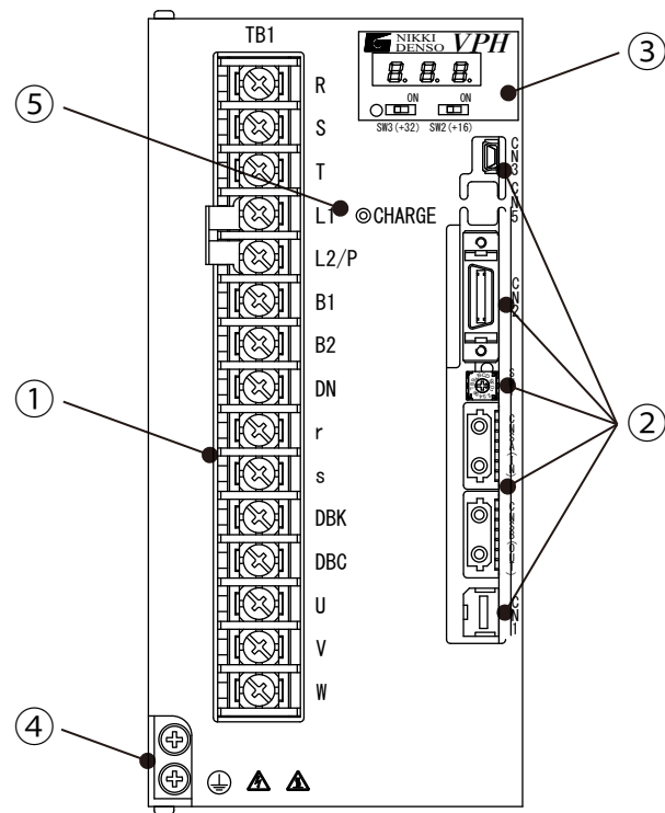
図12-6 1.5kW、2.2kW装置本体正面図 (Type3)
