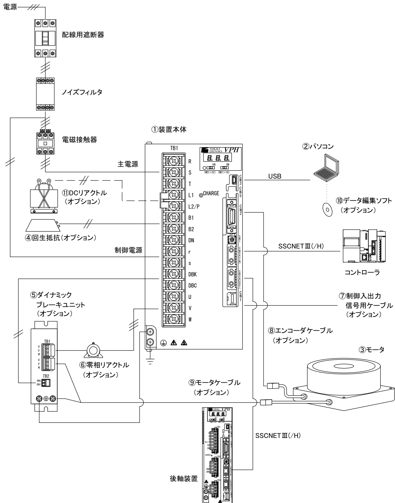
図1-2 1.5kWクラス以上VPH HBタイプ システム構成
