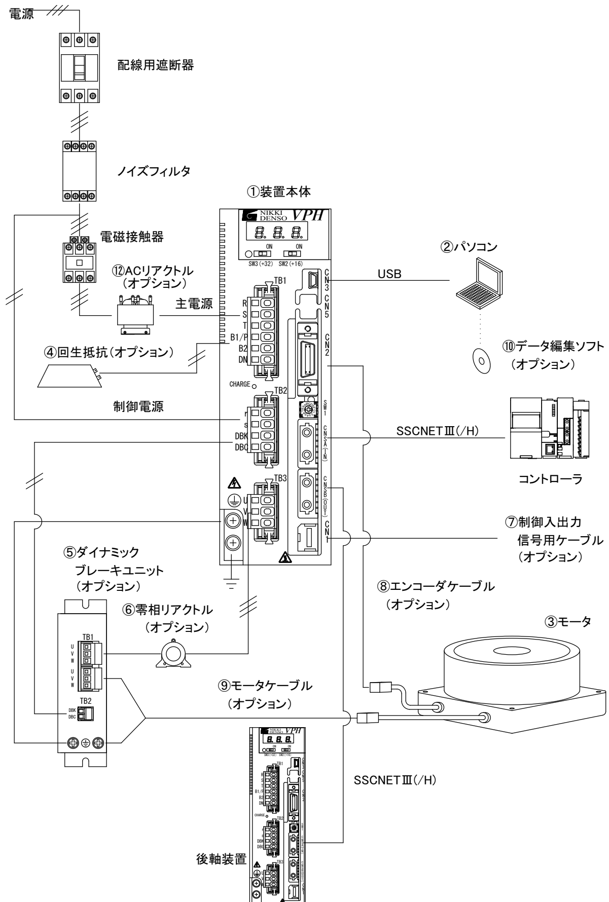
図 1-1 800Wクラス以下 VPH HBタイプ システム構成
