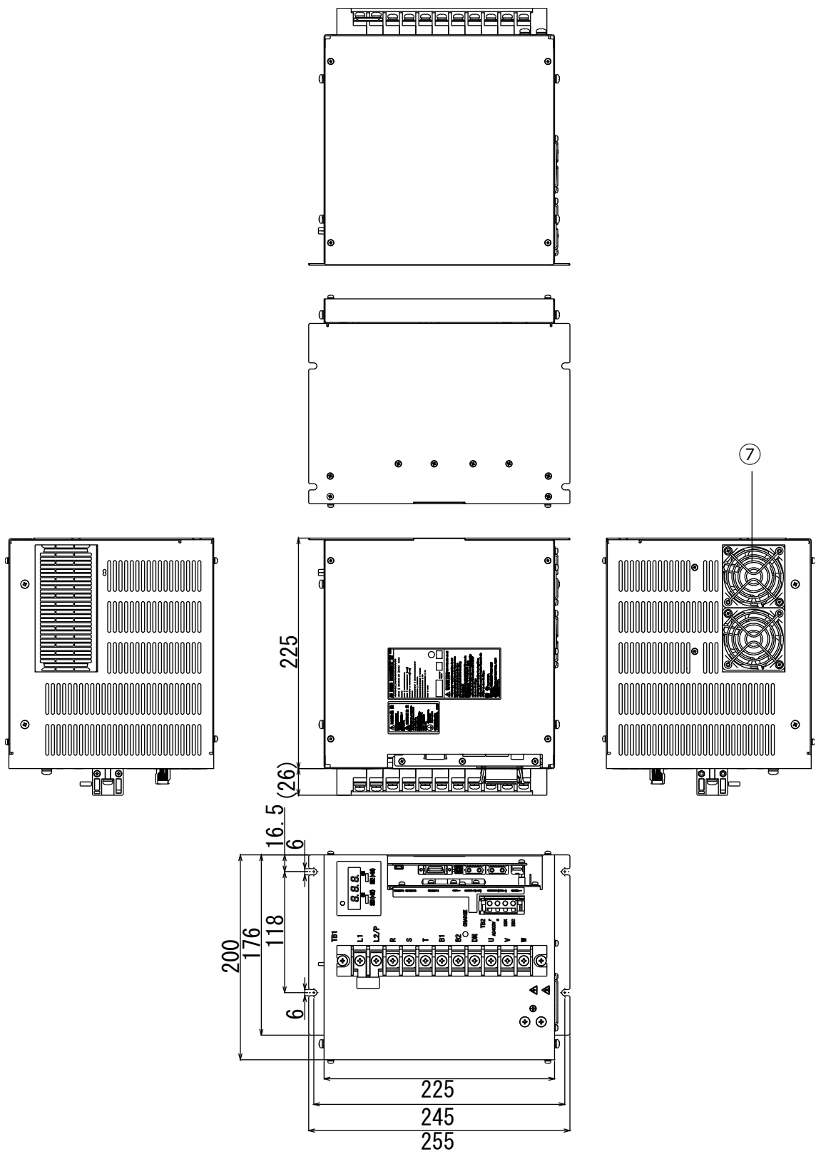
図12-13 400V 7kW装置本体外形図 (Type7)
