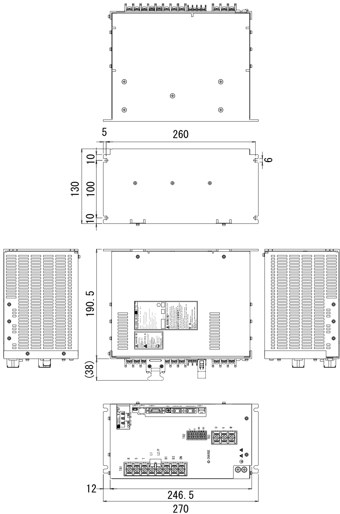
図12-7 3.3kW装置本体外形図 (Type4)
