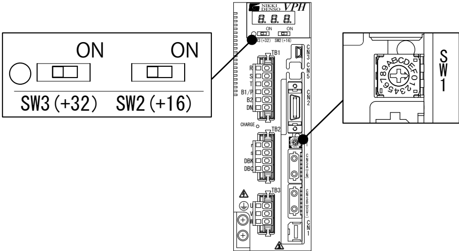
図1-4 制御軸選択スイッチ
