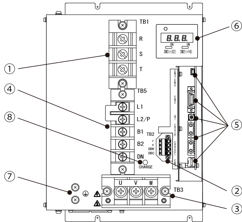
図12-12 15kW装置本体正面図(Type6)
