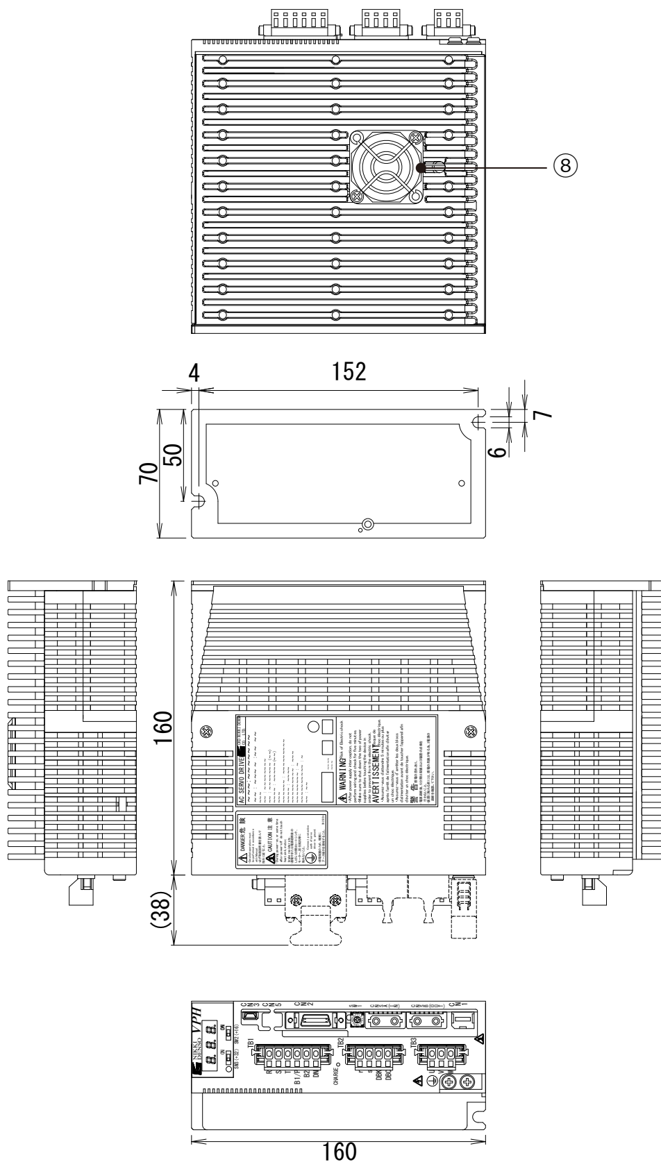
図12-3 800W装置本体外形図 (Type2)
