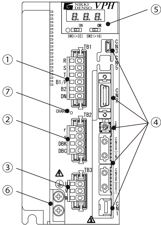
図12-4 800W装置本体正面図 (Type2)
