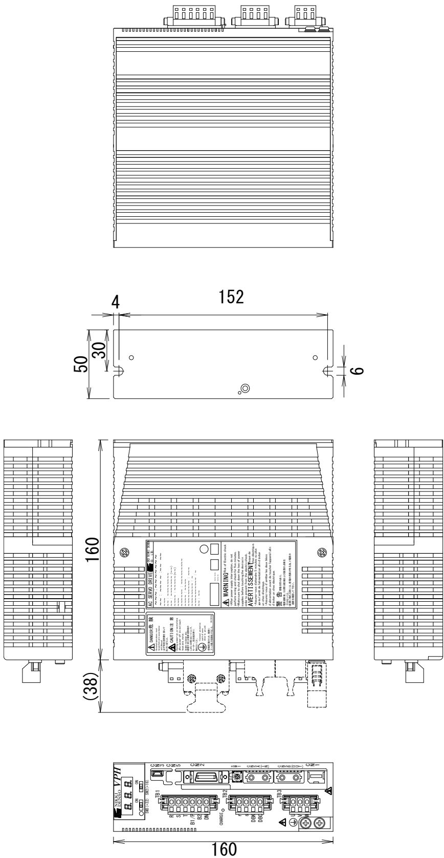
図12-1 400W以下装置本体外形図 (Type1)
