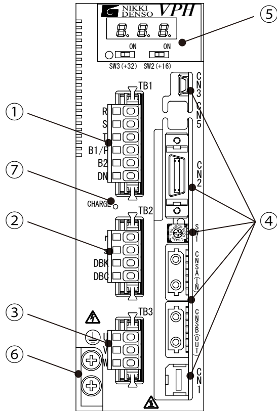
図12-2 400W以下装置本体正面図 (Type1)
