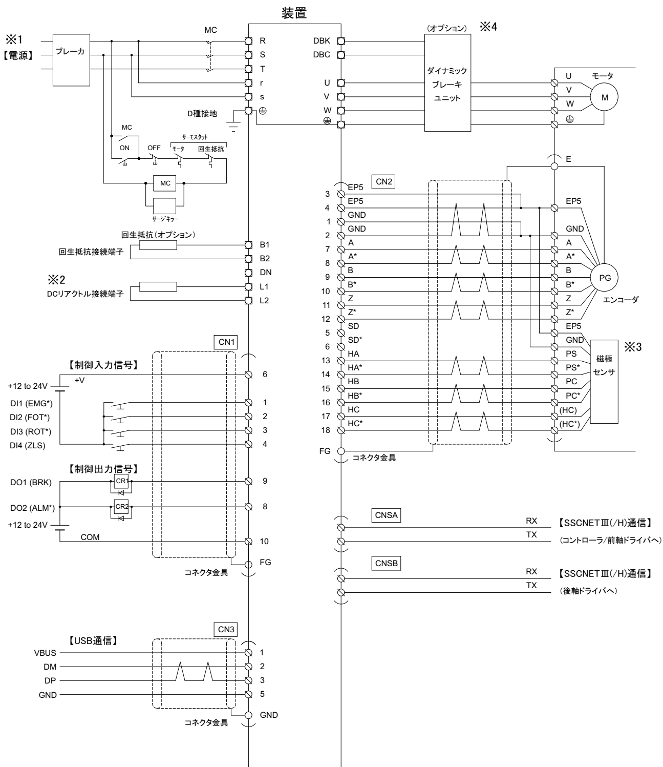
図3-1 外部接続図
