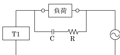
図7・コンデンサ C=0.03~0.1 μF ・抵抗 R=1~3KΩ 岡谷電機製 XEB1K1 又は相当品
