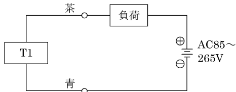
図1 T1 基本回路例
