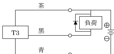
図5 誘導負荷にサージ吸収素子(ダイオード)を使用した例。ダイオードは日立製作所製 V06C、または相当品を使用してください。
