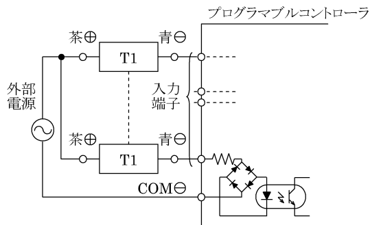
図 11 AC 入力(電源外付)形への T1 接続例
