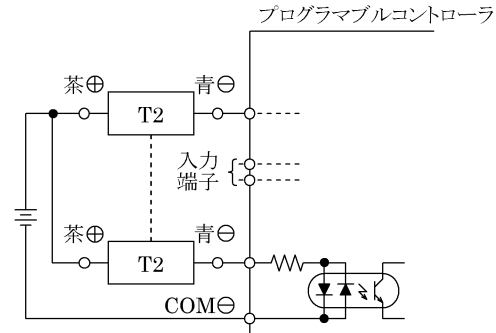
図 14 シンク入力(電源外付)形への T2 接続例
