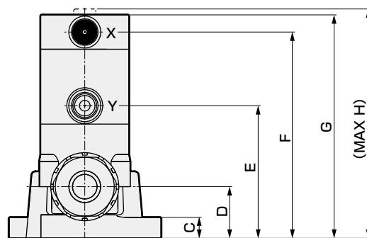
操作ポート方向 (R視図)
