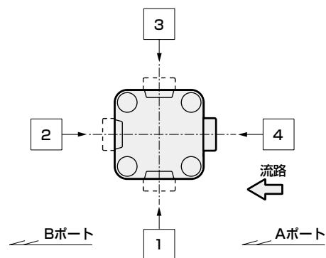
操作ポート方向 (R視図)
