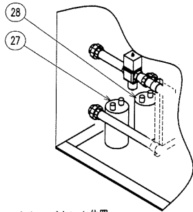
レシーバタンク位置 GT7400WD,GT7480WD
