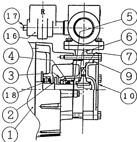
構造 断面図
