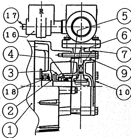
構造 断面図
