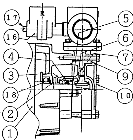
構造 断面図
