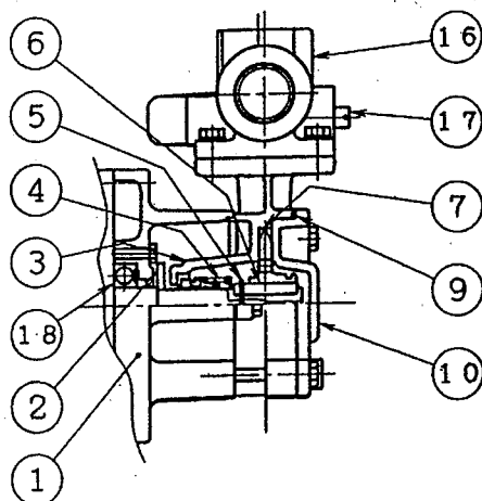
構造 断面図
