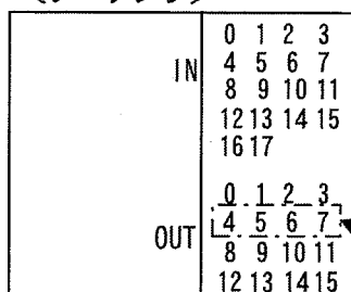
＜シーケンサ＞
